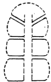
Fig. 23. — Uteria encrinella MICH. — Section longitudinale schématique.
