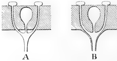
Fig. 9. — Neomeris LAMX, section Vaginopora DEFR. — Sections schématiques de la paroi. A. V. fragilis DEFR. B. V. arenularia MUN.-CH.
