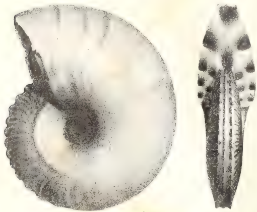
Fig. 11. — Distichoeras bipartitum ZIETEN. Figure de la Paléontologie française, Céph. jur., pl. 158, fig. 1, 2.
