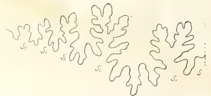
Fig. 32. — Creniceras Rengeri OPPEL. Dives. Éch. figuré pl. I, fig. 18; \times 10 .
