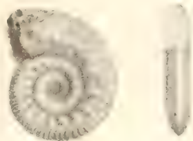
Fig. 6. — Hecticoceras suevum BON. Figure type in : QUENSTEDT, Atlas z. d. Ceph. (1849), pl. VIII, fig. 1, Br. J. ζ, Gammelshausen.
