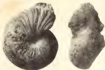
Fig. 13. — (?) Tarmelliceras sp.
