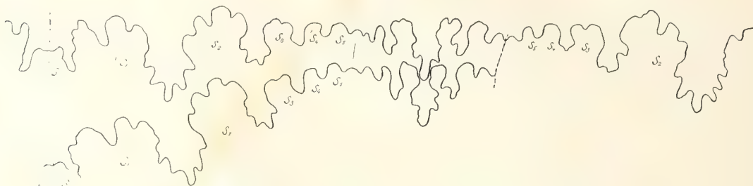
Fig. 21. — Horioceras Baugieri D'ORB. Villers-sur-Mer, H. 1-3; \times 13 .
