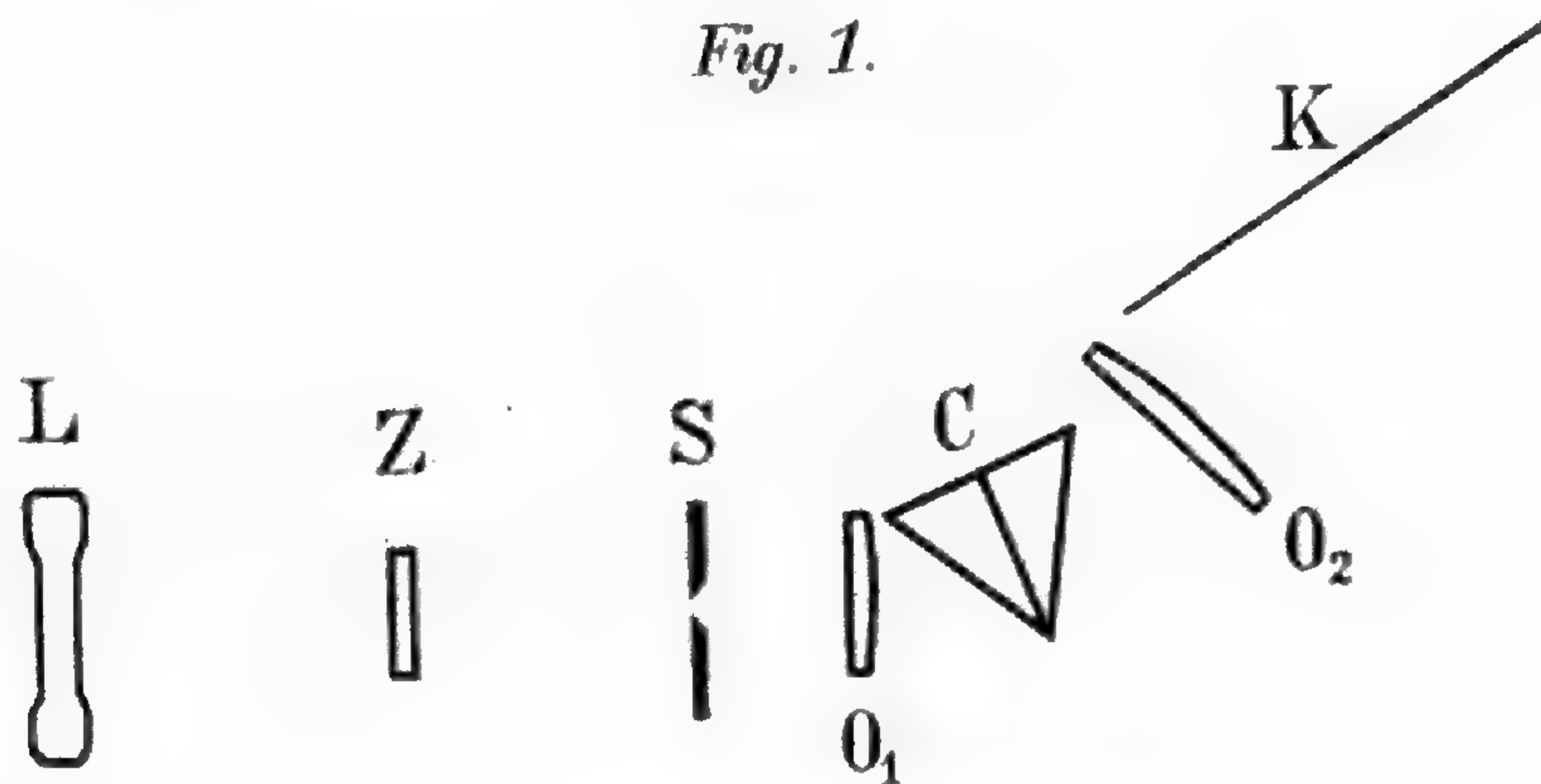
Quarzspektroskop mit Leuchtschirm.
