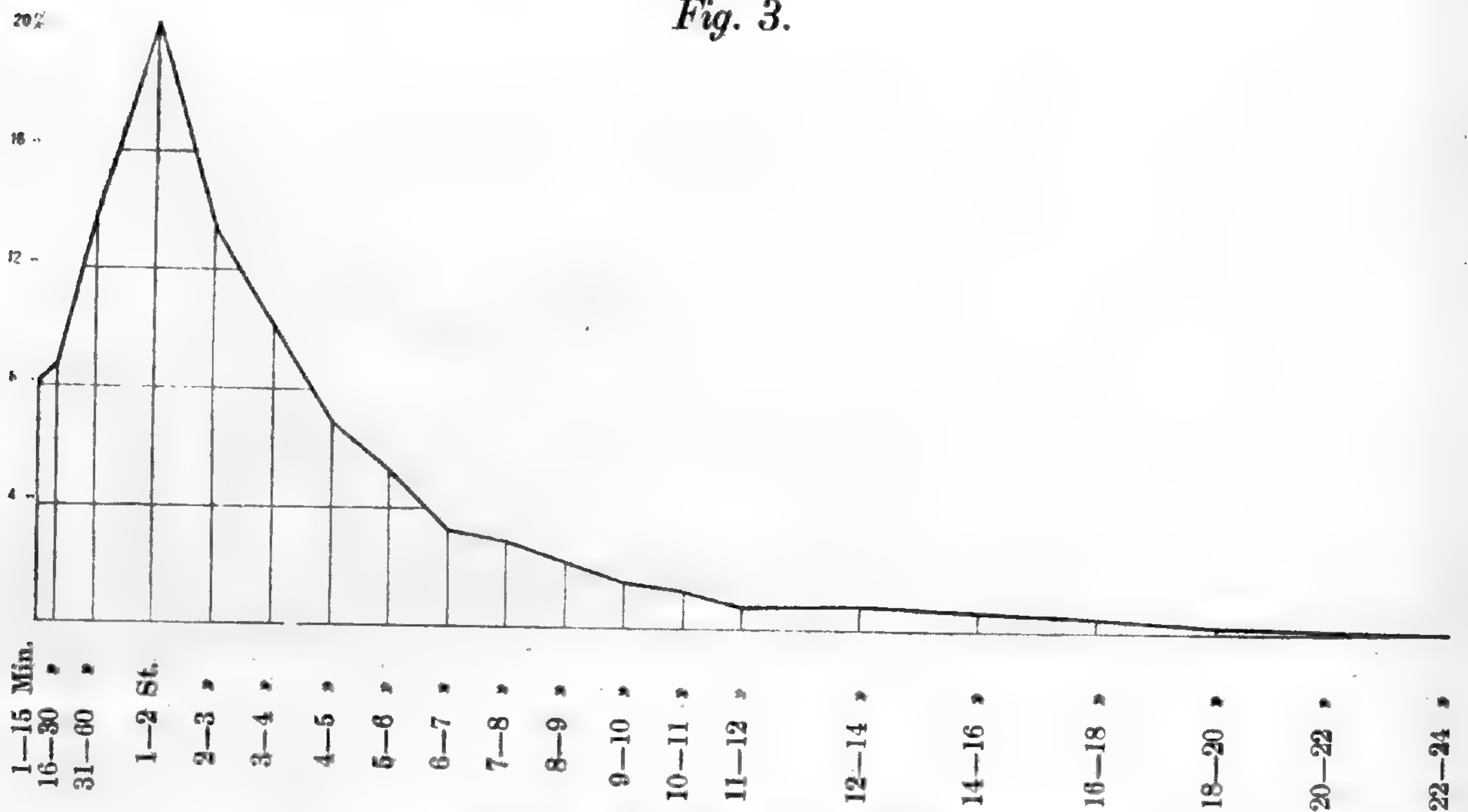
Zahl der Regentage mit verschieden langer Regendauer.
