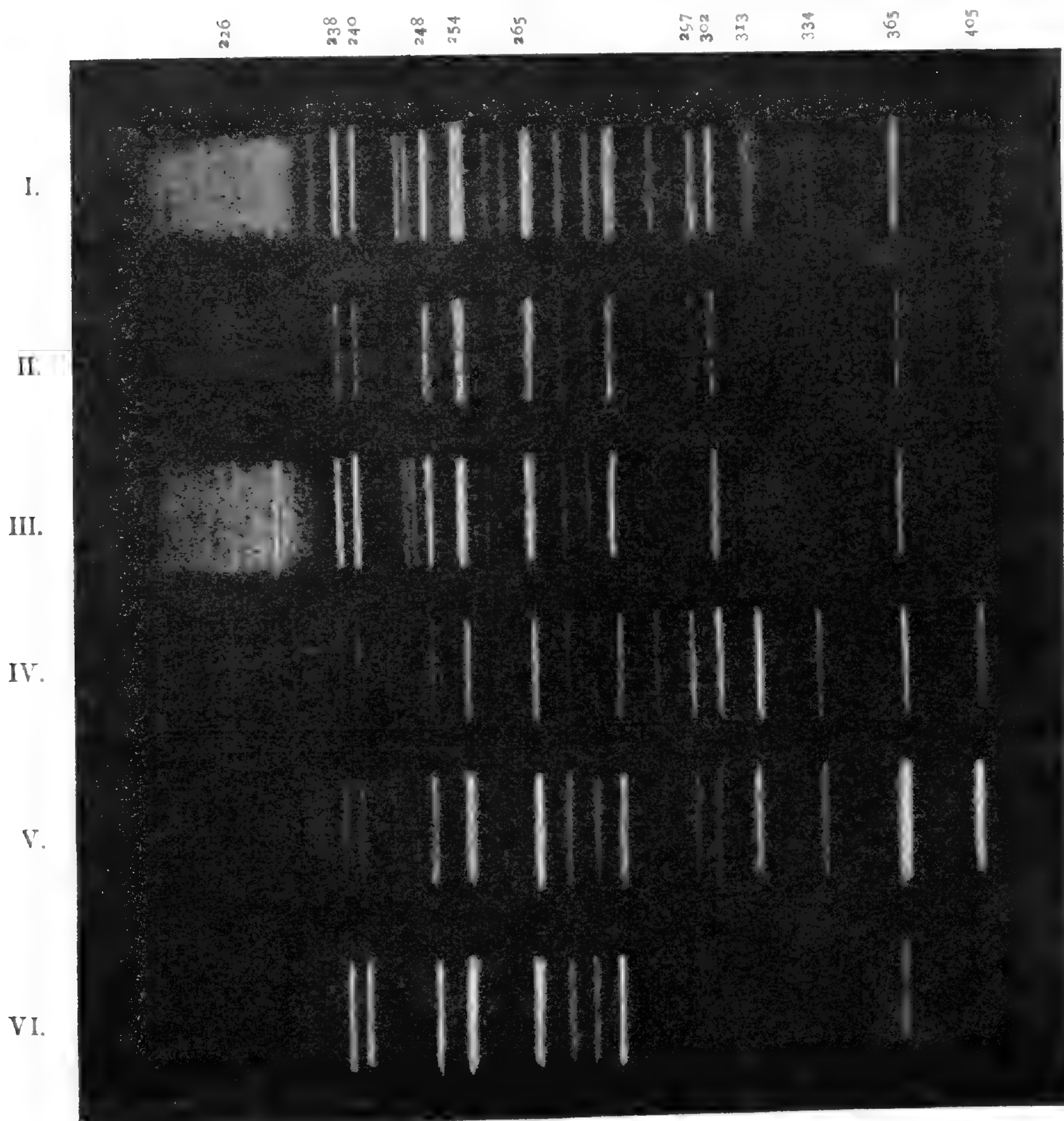
Fluoreszenz durch Belichtung mit dem ultravioletten Spektrum einer Quarzglas-Quecksilberbogenlampe. I. Grüner Troostit. — II Gelber Troostit. — III. Weißer Troostit. — IV. Zinkoxyd. — V. Sodalith aus Grönland. — VI. Tephroit.
