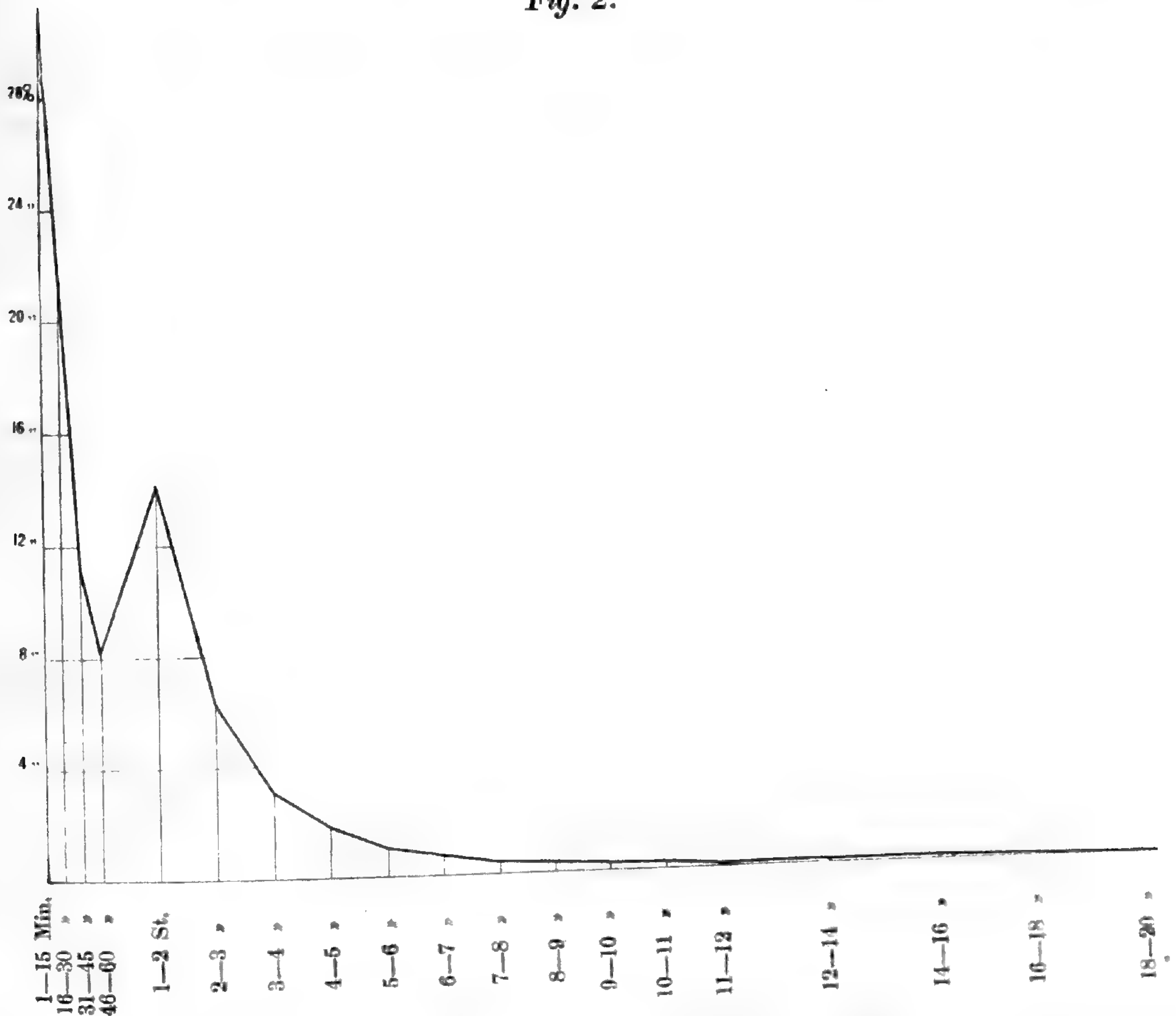
Zahl der Regenfälle von verschieden langer Dauer.
