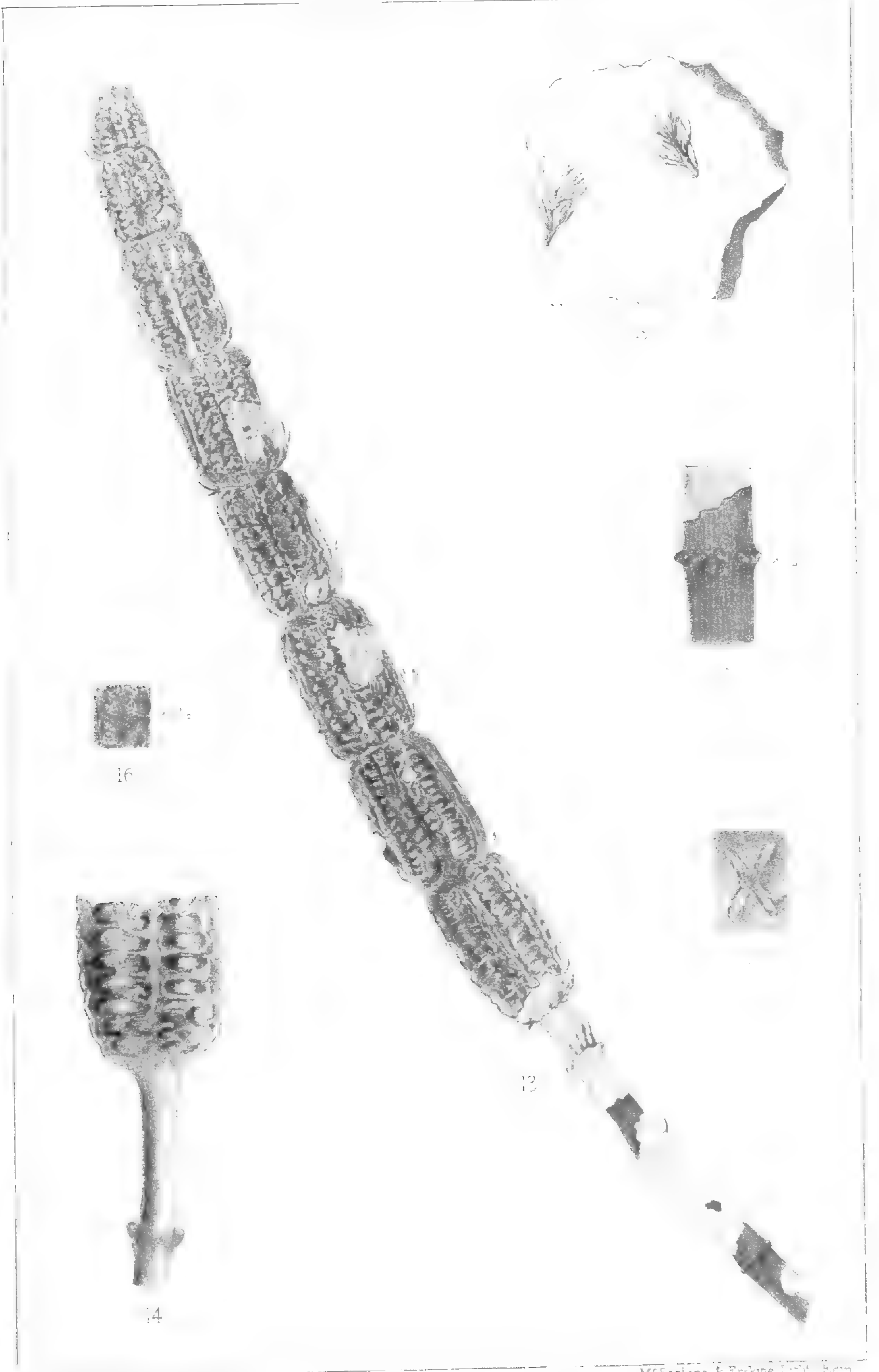
13-17. FRUIT OF BORNIA. Roem. 18. SPHENOPHYLLUM TENERRIMUM. Ett
