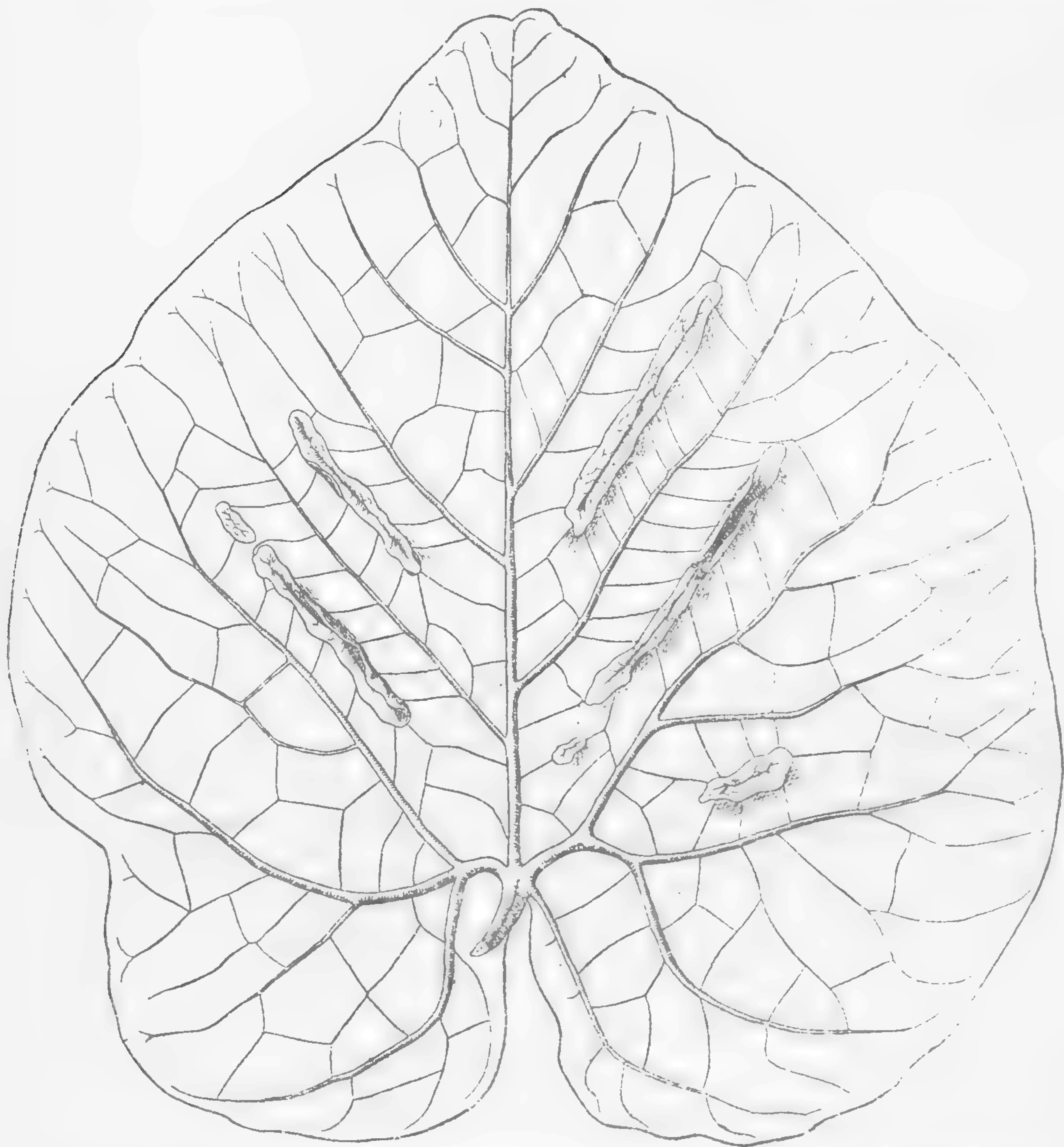
FIG. 1. — Face inférieure d'une feuille d' Aristolochia Siphon , pourvue d'appendices foliacés surnuméraires (1/2 grandeur nat. environ).
