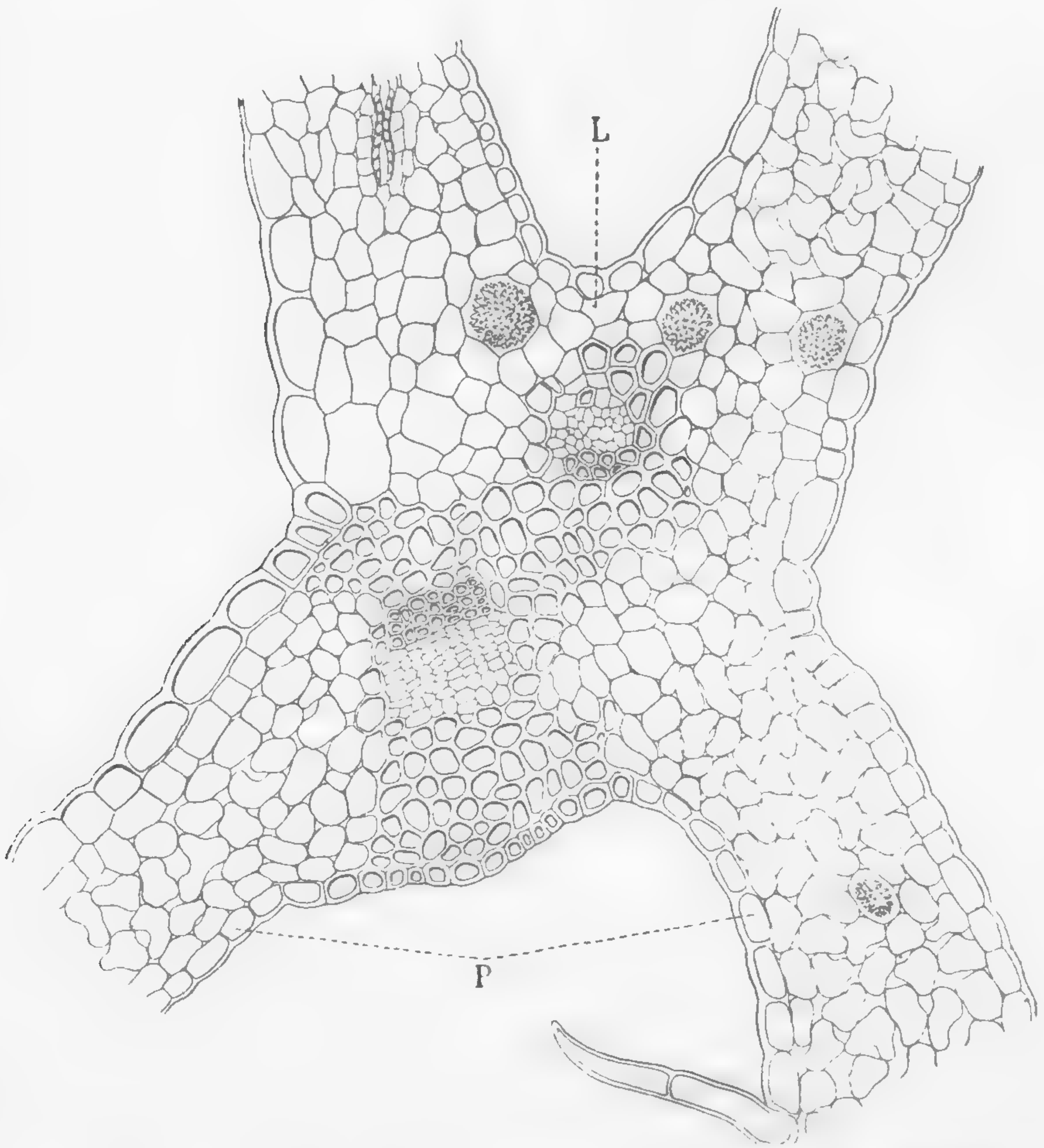
FIG. 3. — Même coupe que dans la figure 2, en montrant les détails histologiques. — Gr. 120 diamètres.
