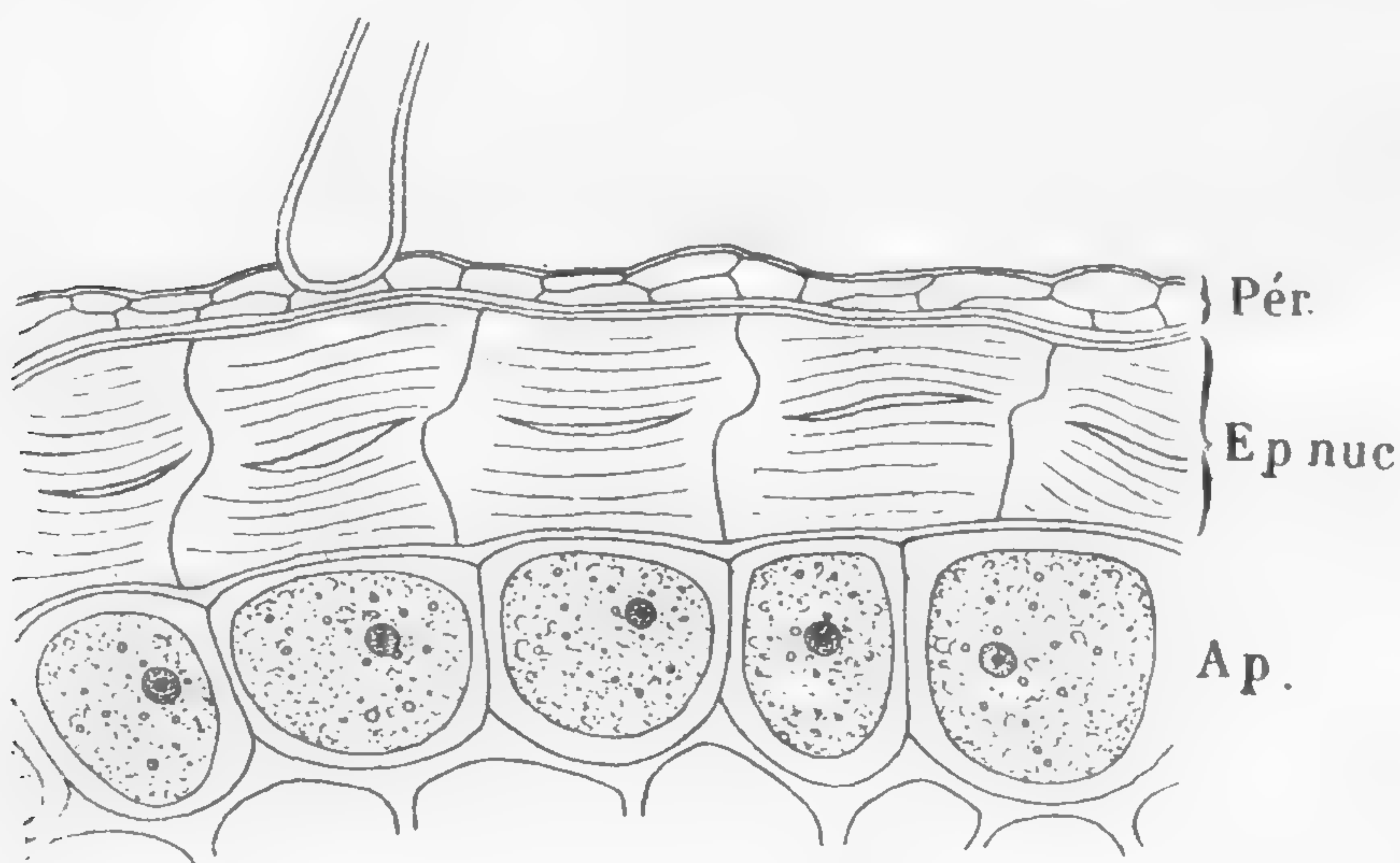
Boissiera bromoides Hochst. — Coupe transversale du caryopse, après traitement à l'eau de Javel et examen dans l'acide lactique. Pér., péricarpe; Ep. nuc., épiderme du nucelle; A. p., assise protéique. Le tégument séminal n'est représenté que par une bande très étroite à structure cellulaire peu distincte. Gr. 480.
