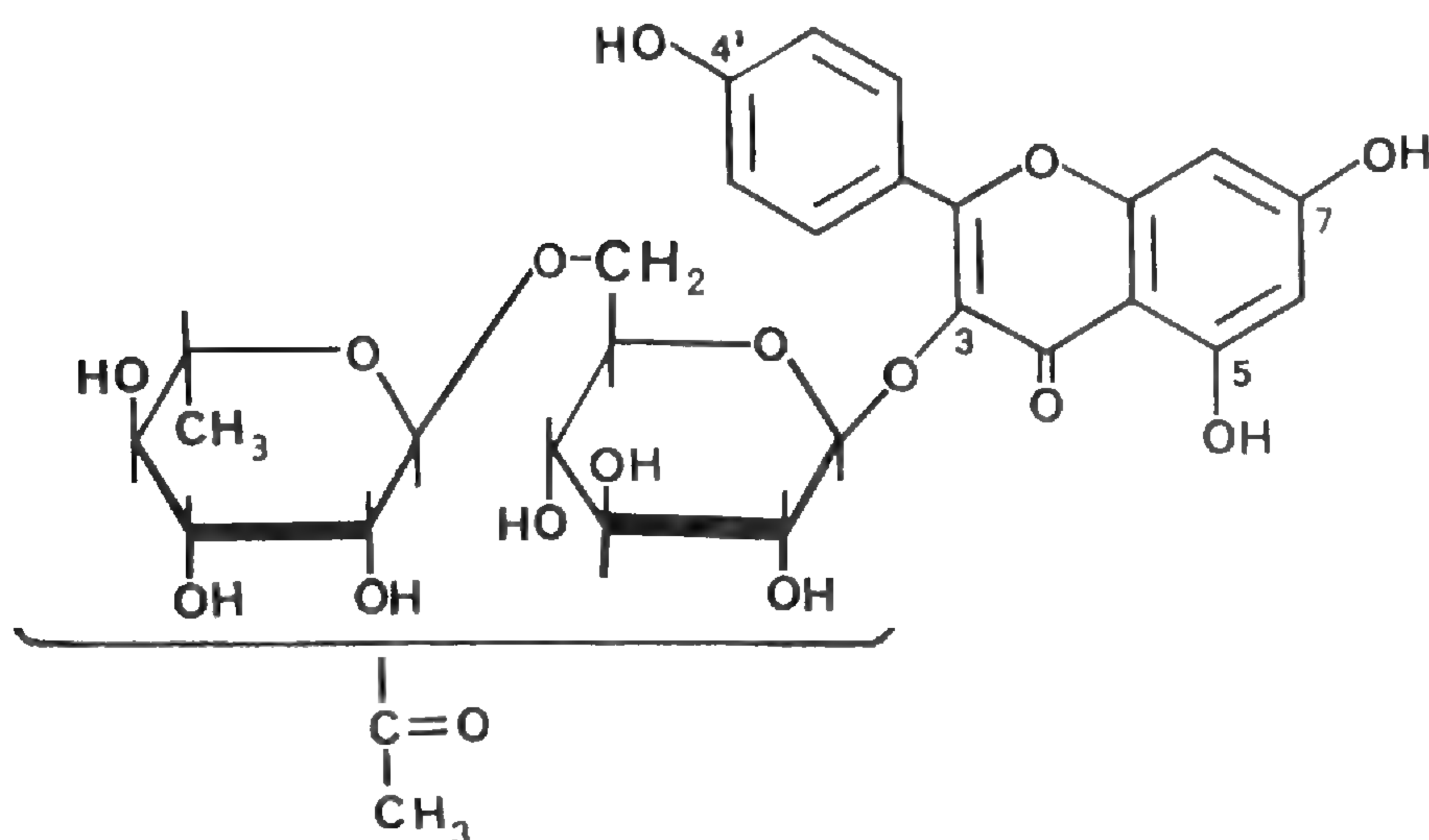
FIG. 1. Kaempferol 3- O -(acetylrutinoside).
