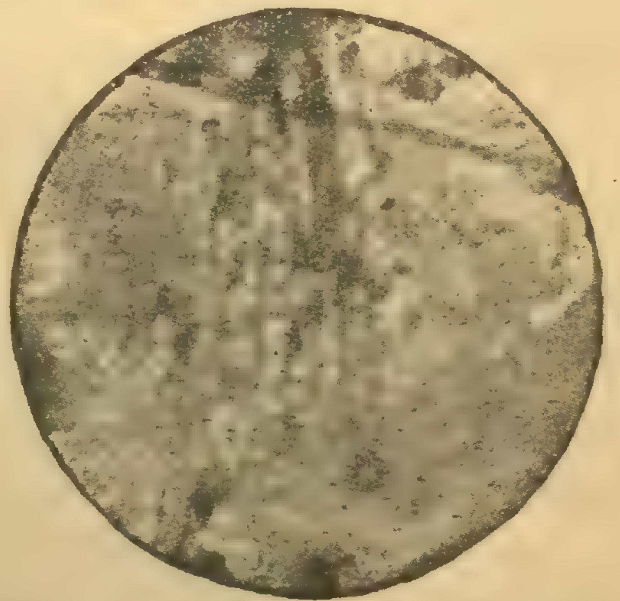
Рис. 6. Kazania elegantissima Stuck. Часть скелетной фибры, съ сильно изъ- ѣденными spicula. Увелич. въ 75 разъ Р. Уфа, противъ дер. Чигвинцевой.
