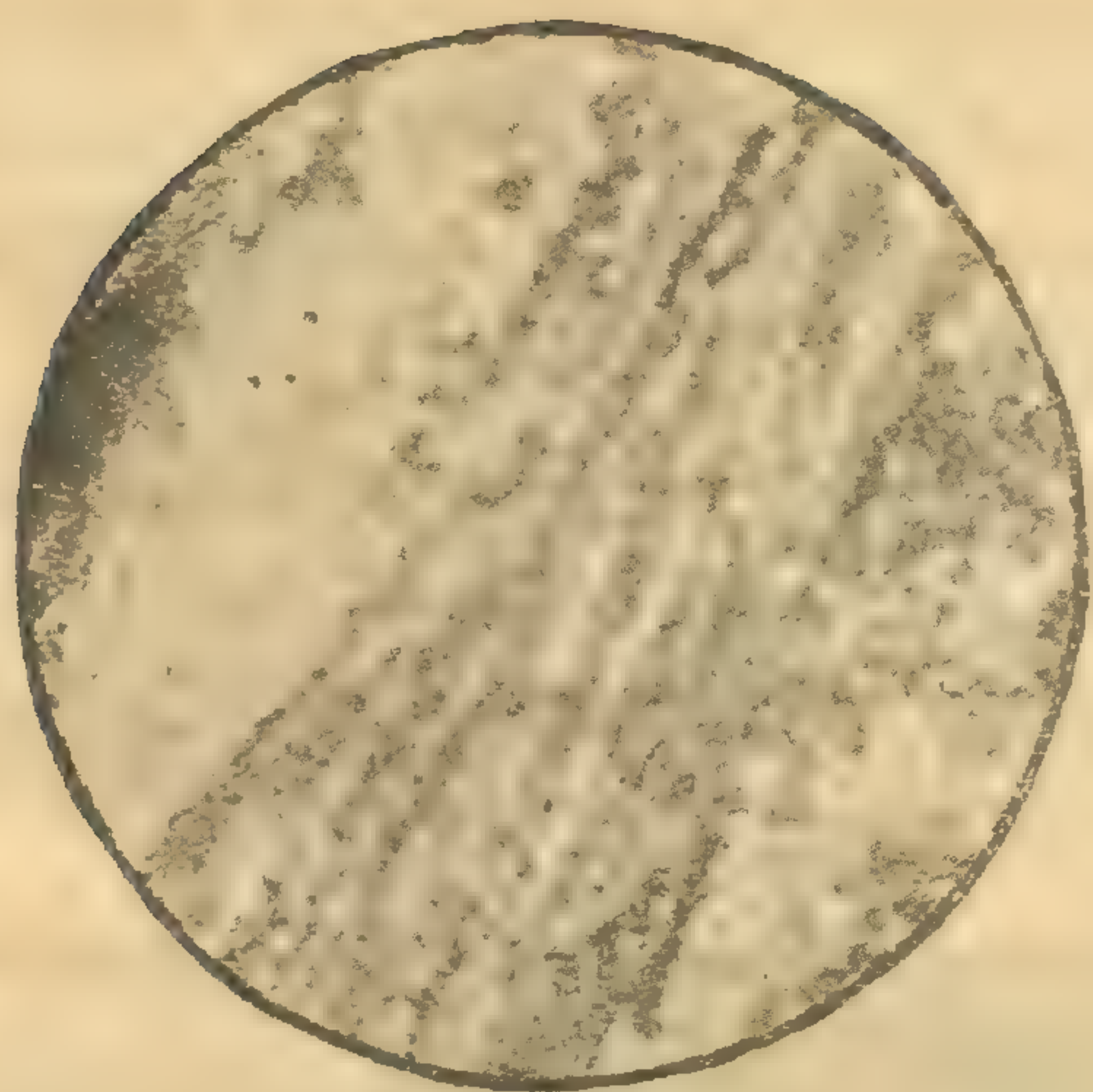
Рис. 8. Kazania elegantissima Stuck. Продольный разрѣзъ фибры. Въ центральной части веретенообразныя и литистидныя spicula, въ периферическихъ частяхъ исключительно литистидныя. Увелич. въ 24 раза. Р. Немь.
