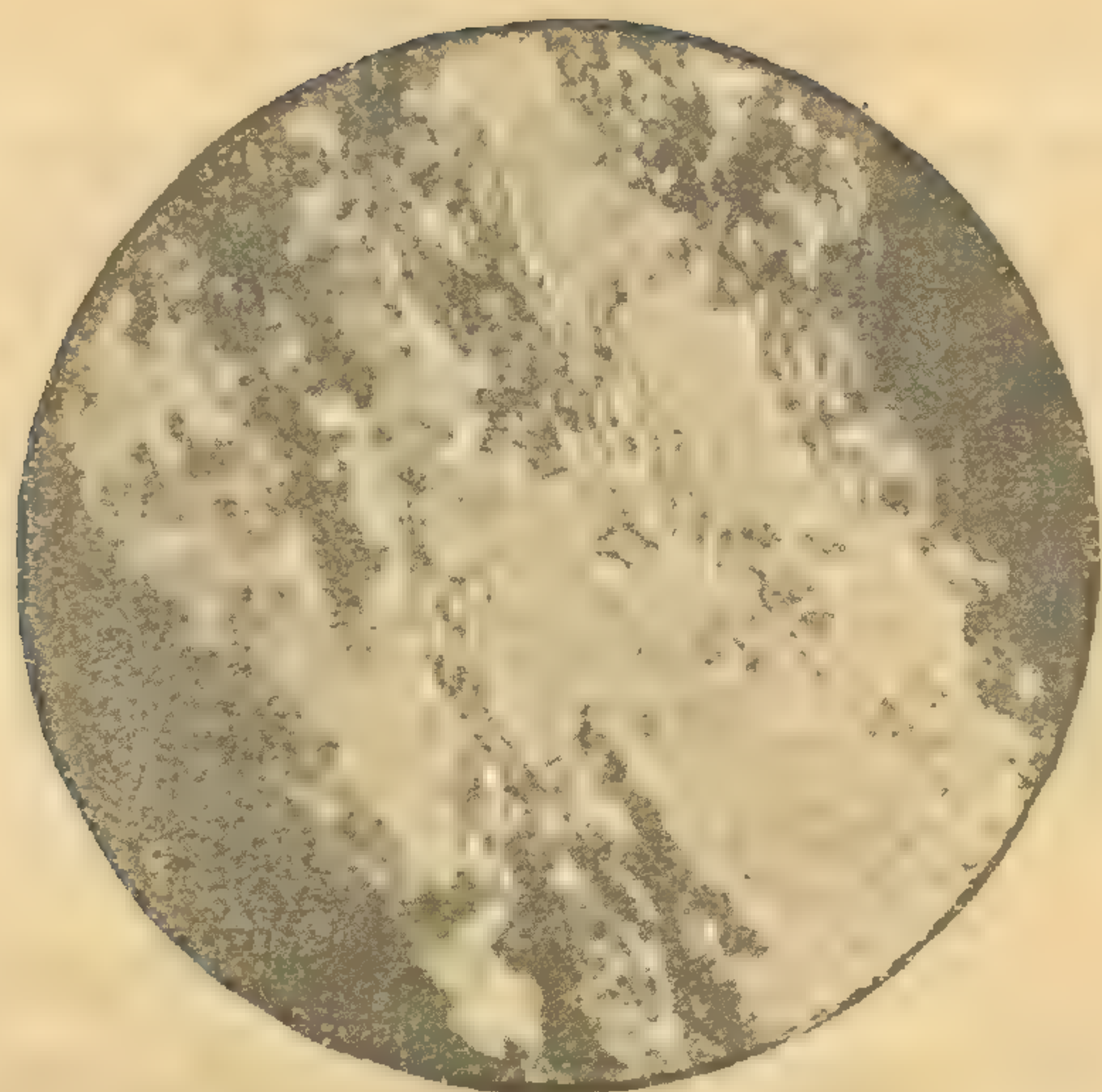
Рис. 9. Kazania elegantissima Stuck. Продольный разрѣзъ фибры, состоящей почти изъ однѣхъ литистидныхъ spicula. Увелич. въ 24 раза. Р. Немь.
