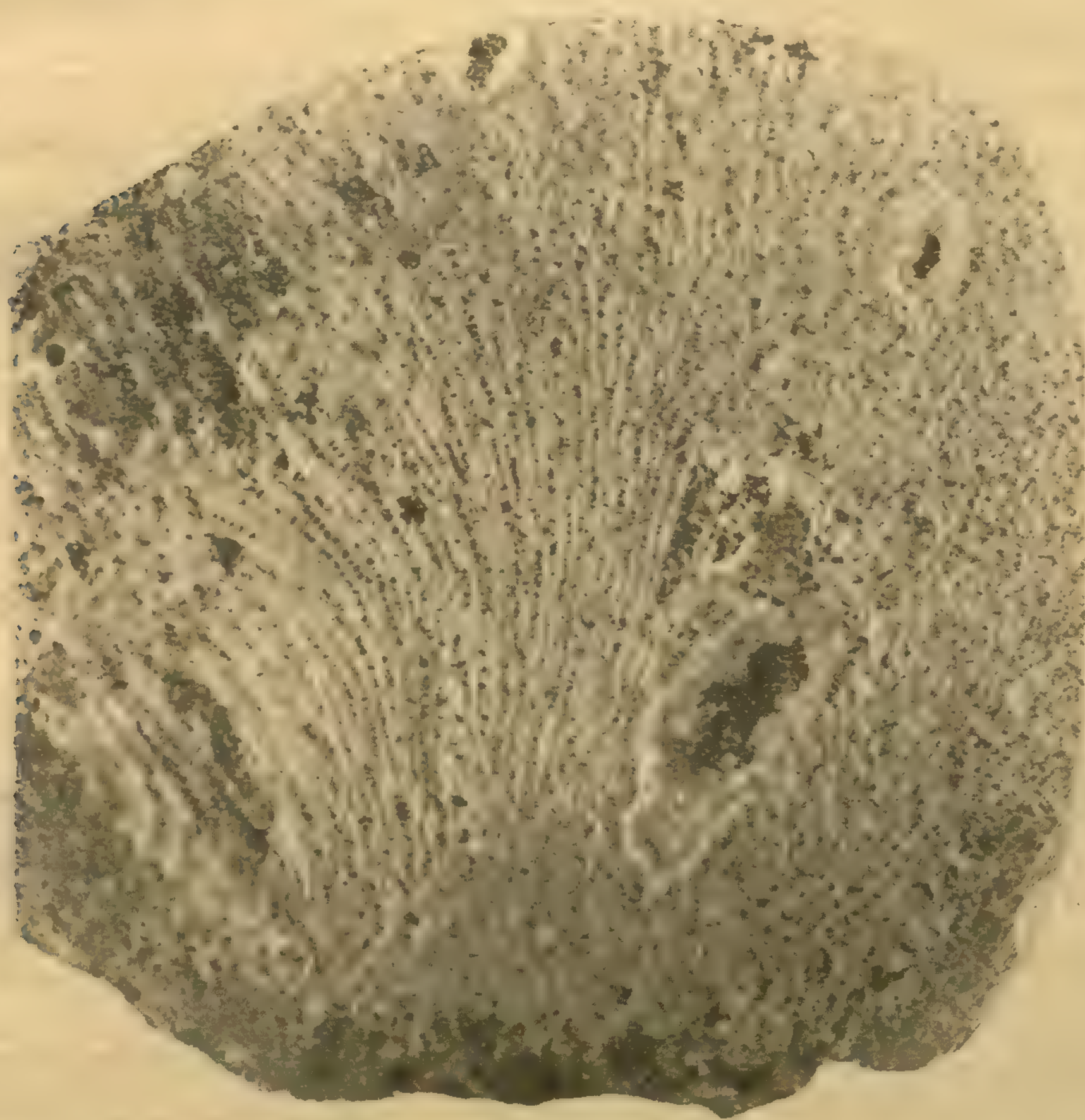
Рис. 13. Stuckenbergia ufensis Stuck. Продольный разрѣзъ скелета, состоящаго изъ рядовъ прутиковъ и спаякъ. Апоризы инкрустированы кварцемъ. Увелич. въ 3 раза. Р. Уфа, противъ дер. Чигвинцевой.
