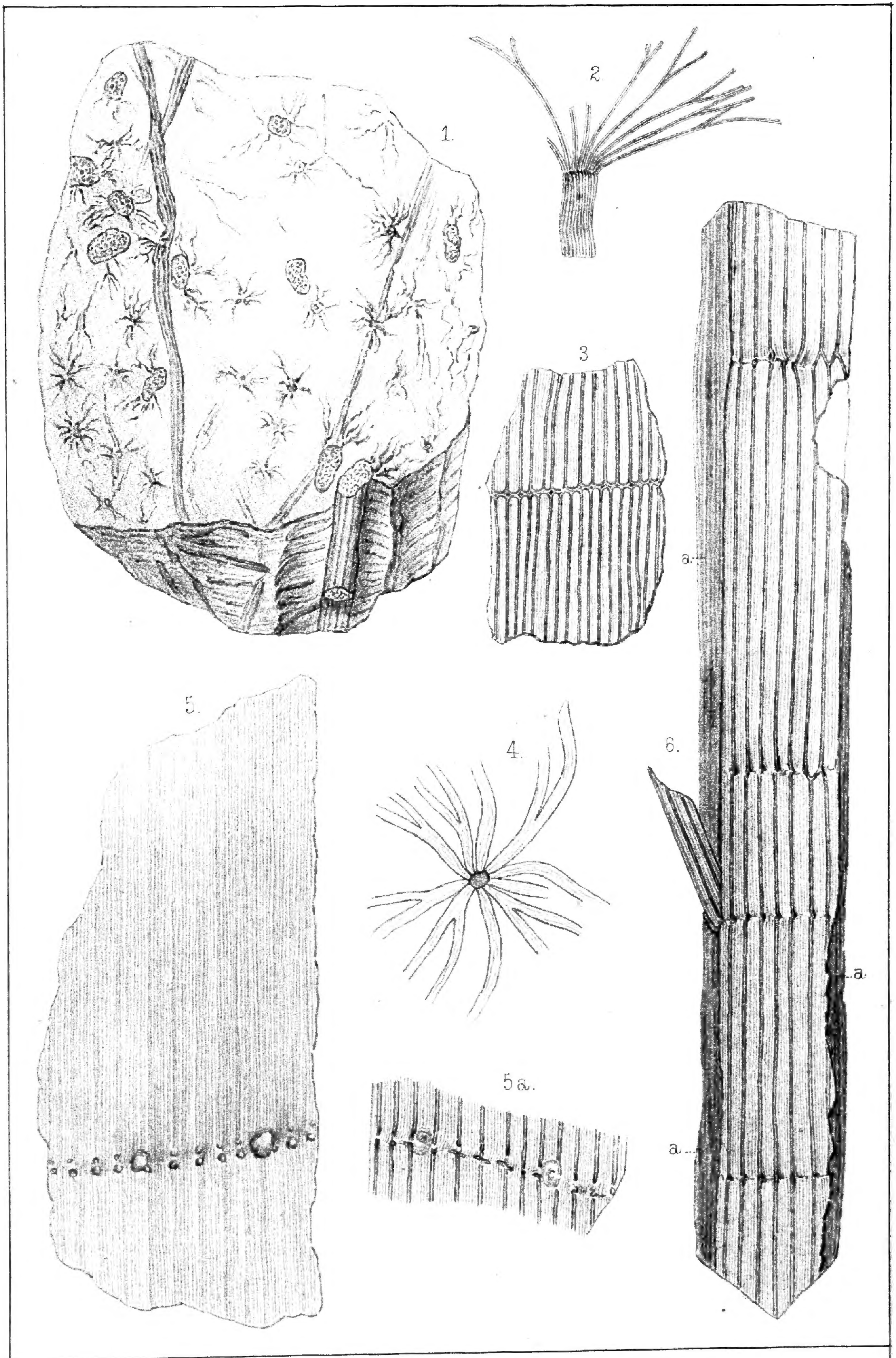
Calamites radiatus.
