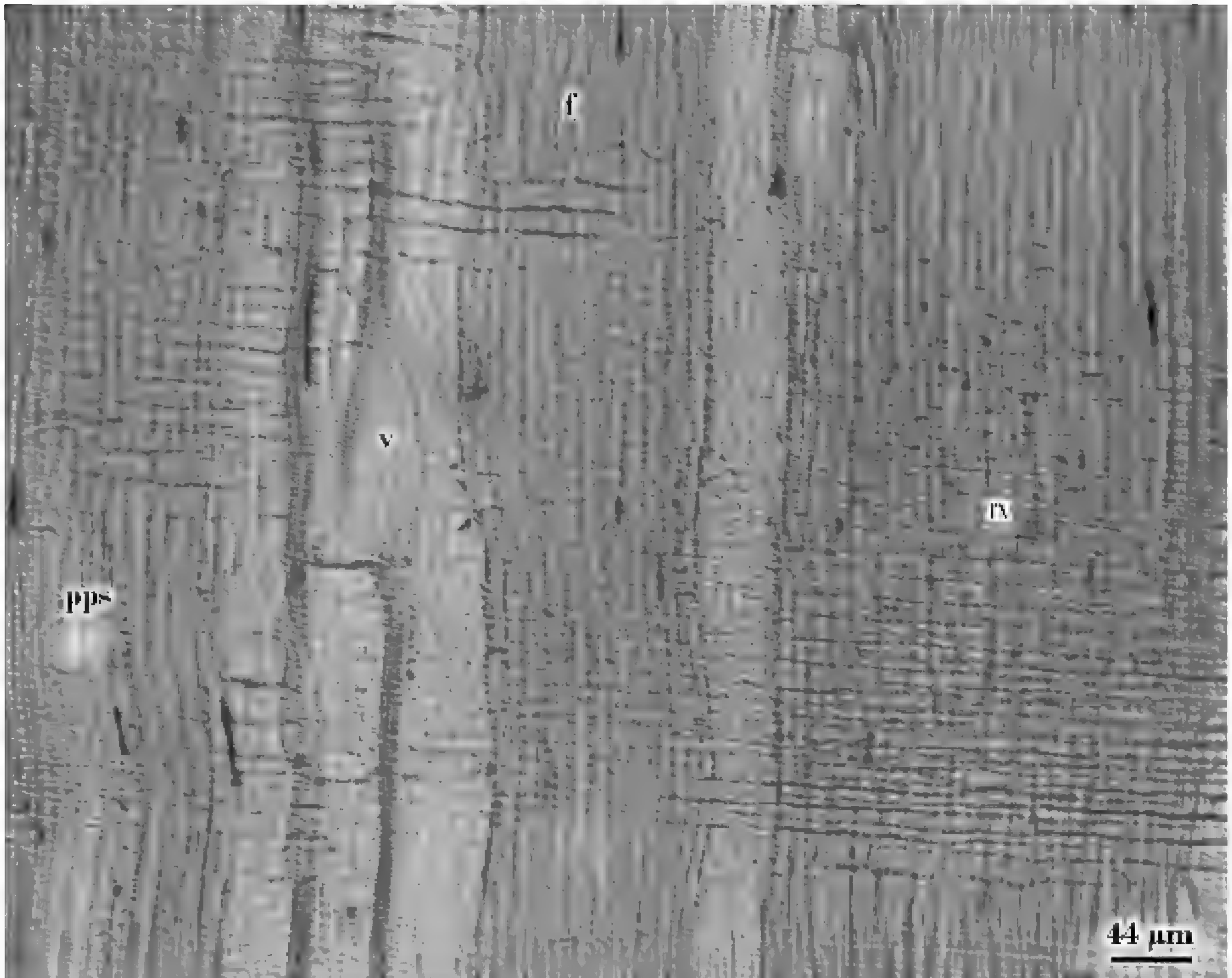
Fig. 100: Leño de Zanthoxylum coco , en corte longitudinal radial. Se observa el largo y alto de los radios, formados por células parenquimáticas procumbentes. El sistema vertical presenta vasos puntuados con placas perforadas simples.
