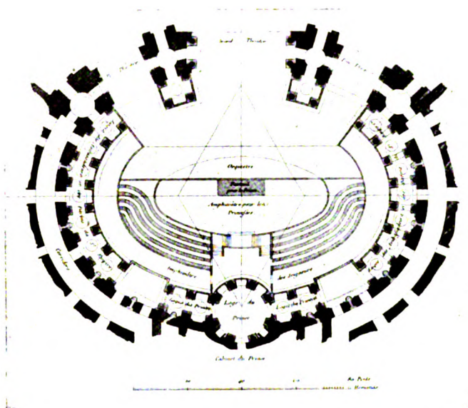
Abb. 14. Dumont: Salles de spectacle. Plan de la nouvelle Salle d'opéra
