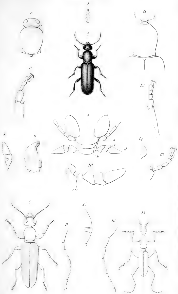
Macrarthrus.
