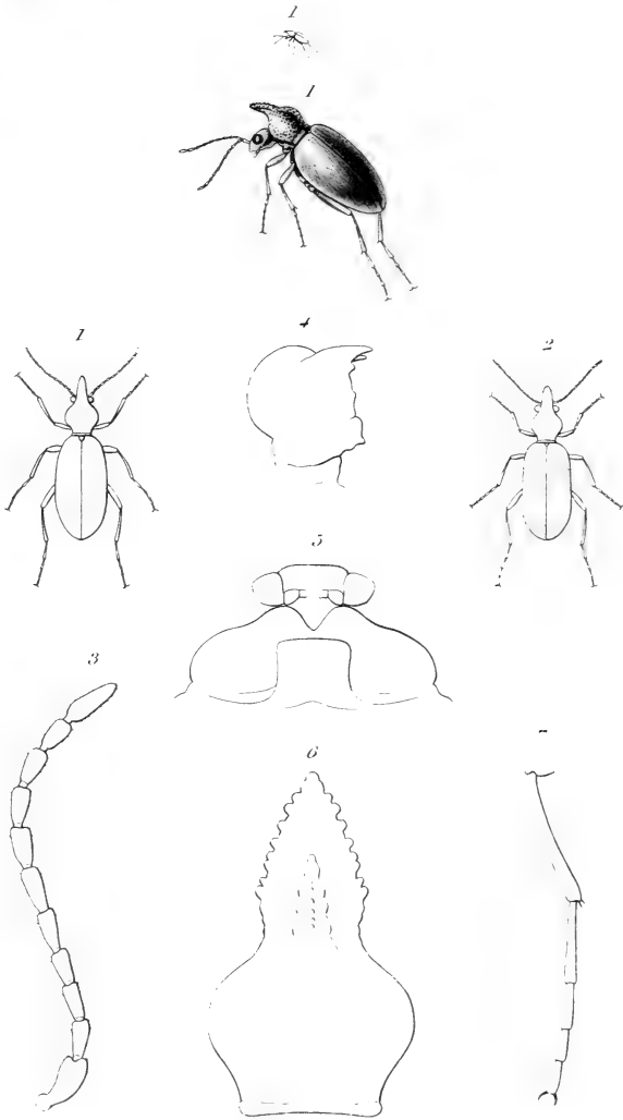
Mecynotarsus.
