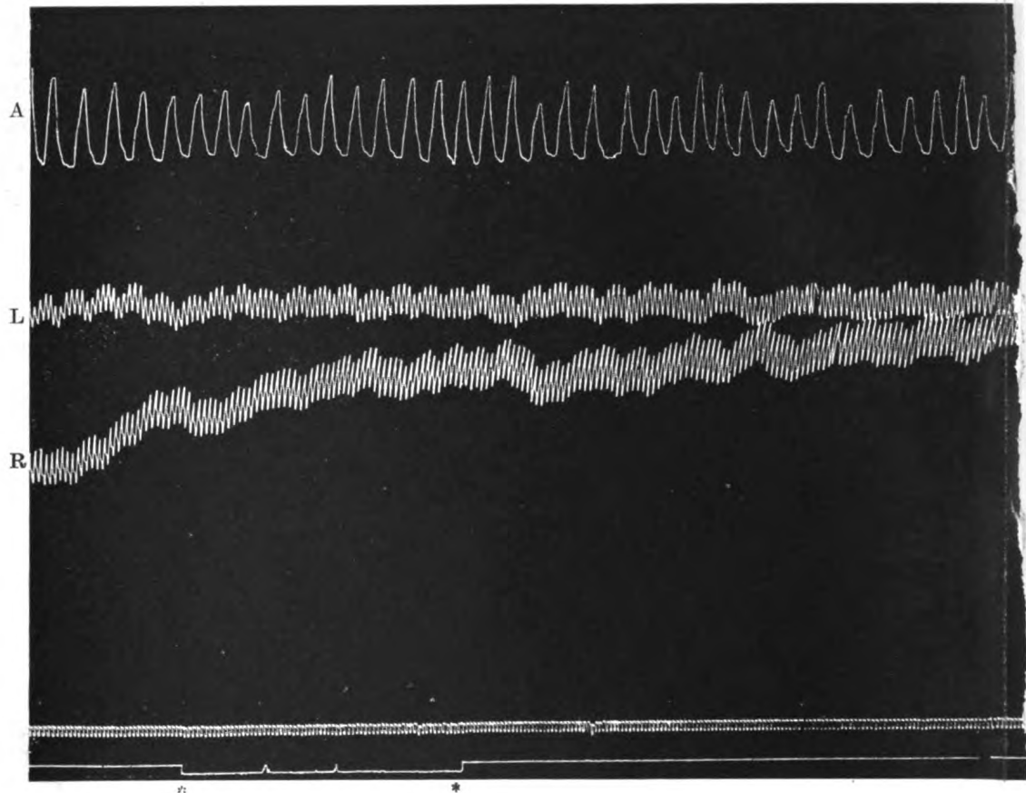
Fall III. Aus Kurve VII. Rechtsseitige Bewegung
