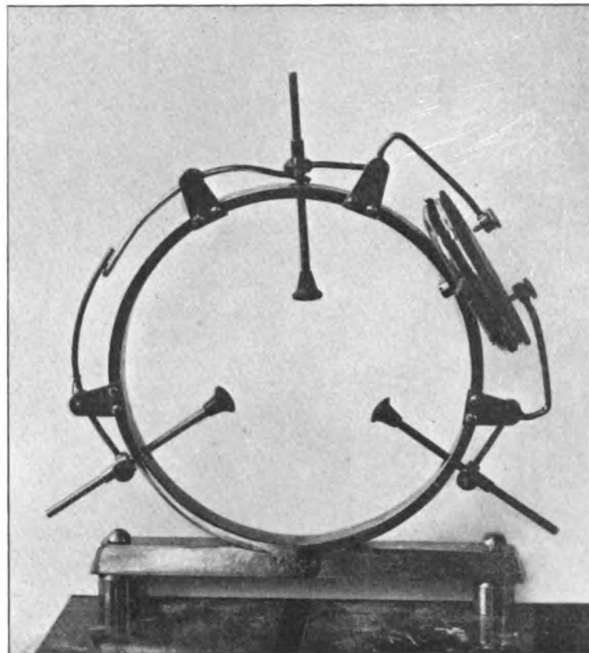
Fig. 7. Kontrollvorrichtung in Vorderansicht.
