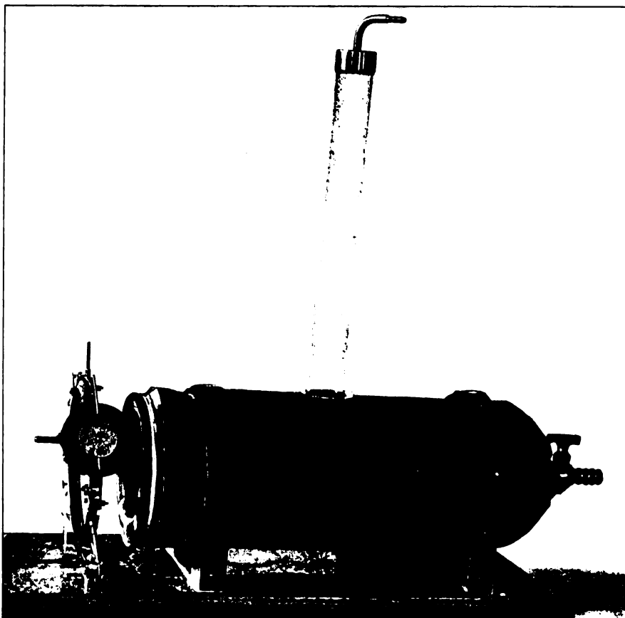
Fig. 8. Kontrollvorrichtung am Plethysmographen in Seitenansicht.
