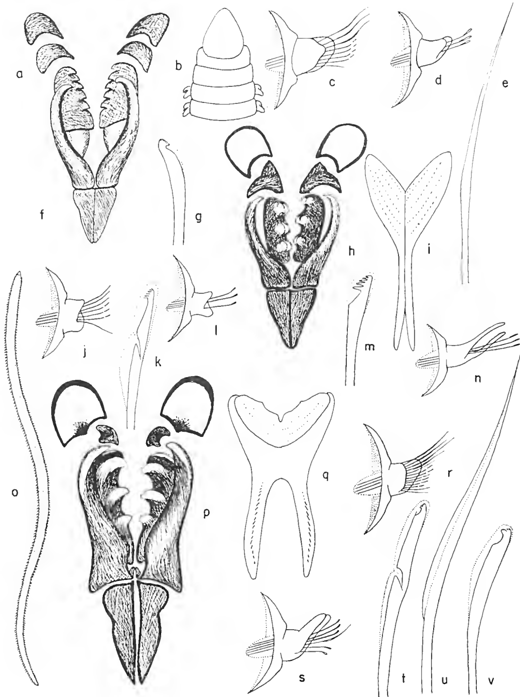
FIG. 17.15. Lumbrineris magalhaensis . (A) Maxillae. (B) Head. (C) Anterior foot. (D) Posterior foot. (E) Capillary seta. (F) Anterior compound hook. (G) Posterior simple hook. Lumbrineris meteorana . (H) Maxillae. (I) Mandibles. (J) Anterior foot. (K) Anterior compound hook. (L) Middle foot. (M) Posterior hook. (N) Far posterior foot. Lumbrineris albidentata . (O) Entire worm (natural size). (P) Maxillae. (Q) Mandibles. (R) Anterior foot. (S) Posterior foot. (T) Anterior compound hook. (U) Capillary seta. (V) Posterior hook.
