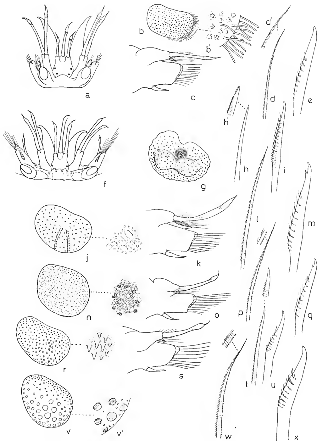
FIG. 1.14. Lepidonotus tenuisetosus . (A) Head. (B) Elytron. (C) Foot. (D) Notoseta. (E) Neuroseta. Lepidonotus cristatus . (F) Head. (G) Fourth elytron. (H) Notoseta. (I) Neuroseta. Lepidonotus glaucus . (J) Elytron. (K) Foot. (L) Notoseta. (M) Neuroseta. Lepidonotus purpureus . (N) Elytron. (O) Foot. (P) Notoseta. (Q) Neuroseta. Lepidonotus semitectus . (R) Third elytron. (S) Foot. (T) Notoseta. (U) Neuroseta. Lepidonotus durbanensis . (V) Third elytron. (W) Notoseta. (X) Neuroseta.
