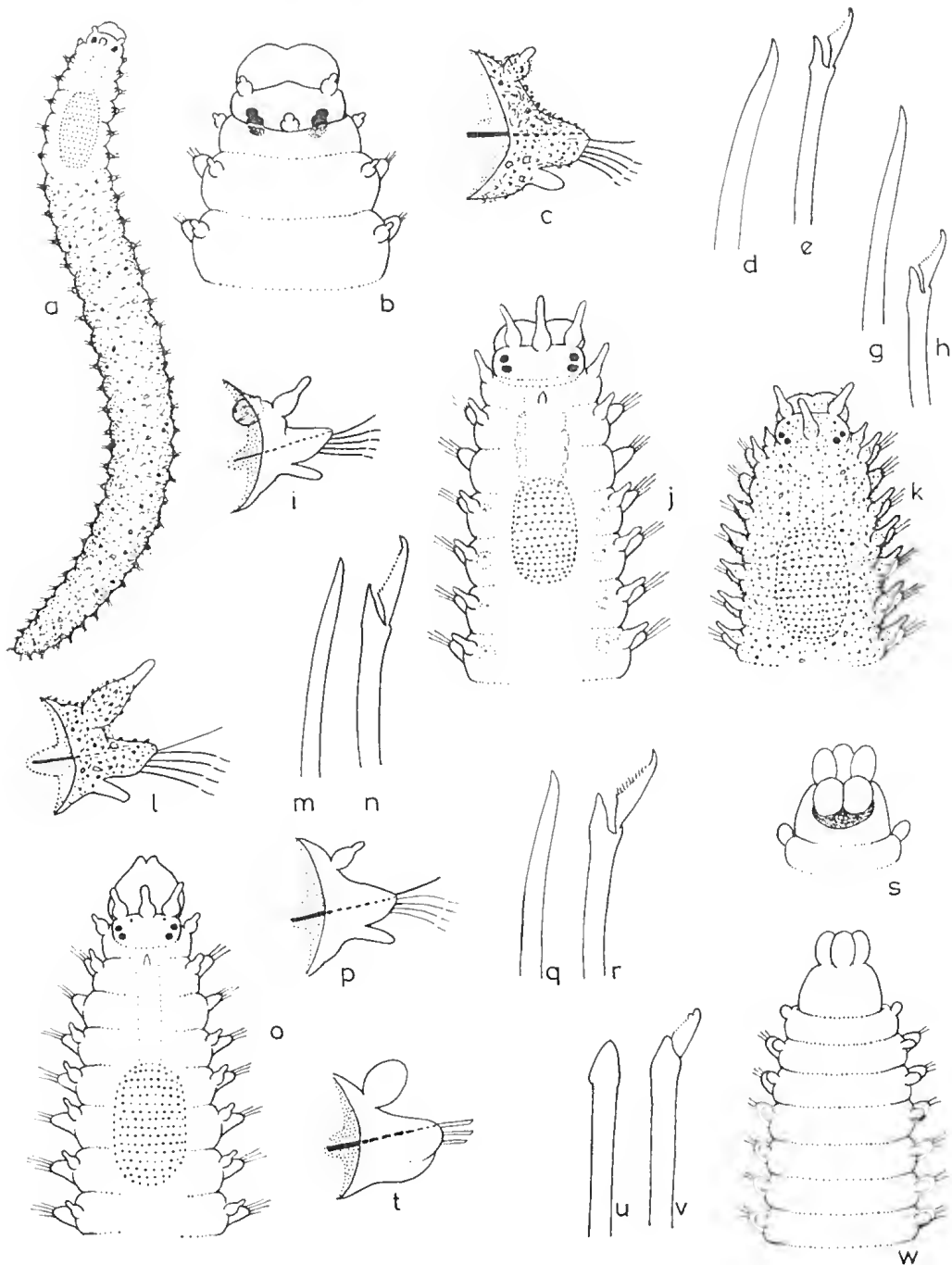
FIG. 12.11. Sphaerosyllis semiverrucosa . (A) Entire worm (20 times life size). (B) Head. (C) Middle foot. (D) Superior simple seta. (E) Compound seta. Sphaerosyllis capensis . (G) Superior simple seta. (H) Compound seta. (I) Middle foot. (J) Anterior end. Sphaerosyllis erinaceus . (K) Anterior end. (L) Foot. (M) Superior simple seta. (N) Compound seta. Sphaerosyllis sublaevis . (O) Anterior end. (P) Foot. (Q) Superior simple seta. (R) Compound seta. Exogonoides antennata . (S) Ventral view of head. (T) Middle foot. (U) Simple seta. (V) Compound seta from anterior foot. (W) Anterior end.
