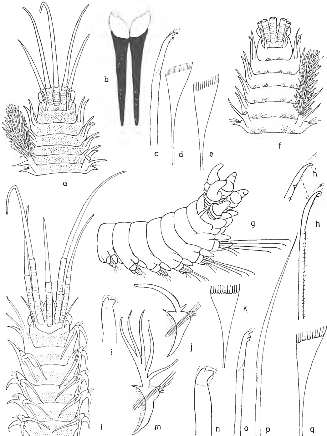
FIG. 17.12. Diopatra cuprea . (A) Anterior end. (B) Mandibles. (C) Pseudocompound seta. (D) Comb seta. Diopatra cuprea punctifera . (E) Comb seta. (F) Anterior end (ceratostyles omitted). Rhamphobrachium capense . (G) Lateral view of anterior end. (H, H 1 ) Pseudocompound seta and variation. (I) Acicular seta. (J) Thirtieth foot. (K) Comb seta. Onuphis erenita . (L) Anterior end. (M) Thirtieth foot. (N) Acicular seta. (O) Pseudocompound seta. (P) Winged capillary. (Q) Comb seta.
