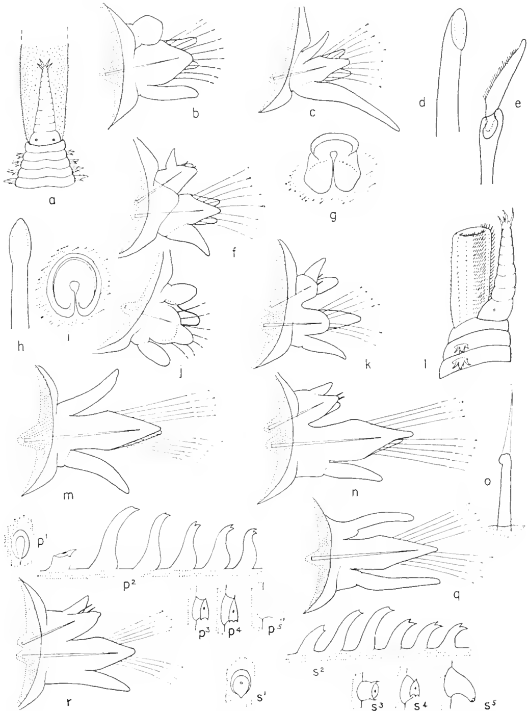
FIG. 16.5. Goniadopsis incerta . (A) Head. (B) Posterior view of anterior foot. (C) Posterior view of middle foot. (D) Acicular notoseta. (E) Falcigerous neuroseta. (F) Posterior view of posterior foot. (G) Proboscideal papilla. Goniadopsis maskallensis . (H) Acicular notoseta. (I) Proboscideal papilla. (J) Posterior view of anterior foot. (K) Posterior view of posterior foot. Glycinde kameruniana . (L) Head with proboscis partly extruded. (M) Anterior view of anterior foot. (N) Anterior view of posterior foot. (O) Acicular notoseta. (P 1-5 ) Proboscideal papillae. Glycinde capensis . (Q) Anterior view of anterior foot. (R) Anterior view of posterior foot. (S 1-5 ) Proboscideal papillae.
