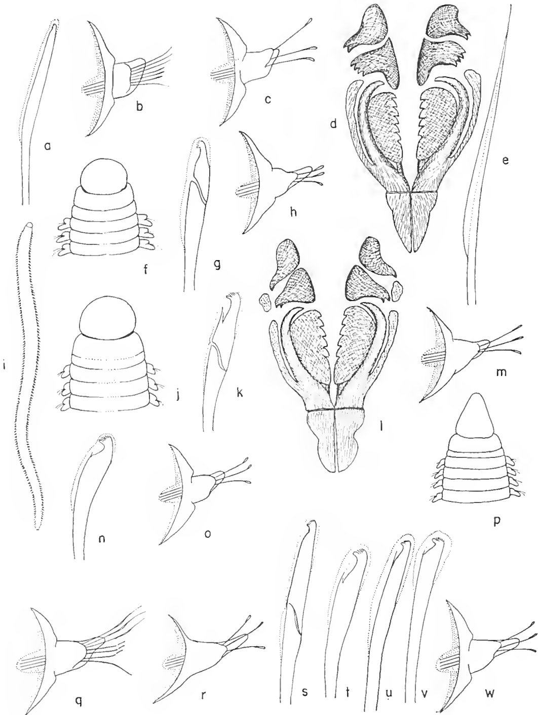
FIG. 17.16. Lumbrineris brevicirra . (A) Anterior hook. (B) Anterior foot. (C) Posterior foot. Lumbrineris inflata (based on a specimen from North Carolina). (D) Maxillae. (E) Capillary seta. (F) Head. (G) Anterior compound hook. (H) Posterior foot. Lumbrineris coccinea . (I) Entire worm (2.5 times life size). (J) Head. (K) Anterior compound hook. (L) Maxillae. (M) Posterior foot. Lumbrineris cavifrons . (N) Anterior simple hook. (O) Posterior foot. Lumbrineris latreilli . (P) Head. (Q) Anterior foot. (R) Posterior foot. (S) Anterior compound hook. (T) Posterior simple hook. Lumbrineris tetraura . (U) Anterior hook. (V) Posterior hook. (W) Posterior foot.
