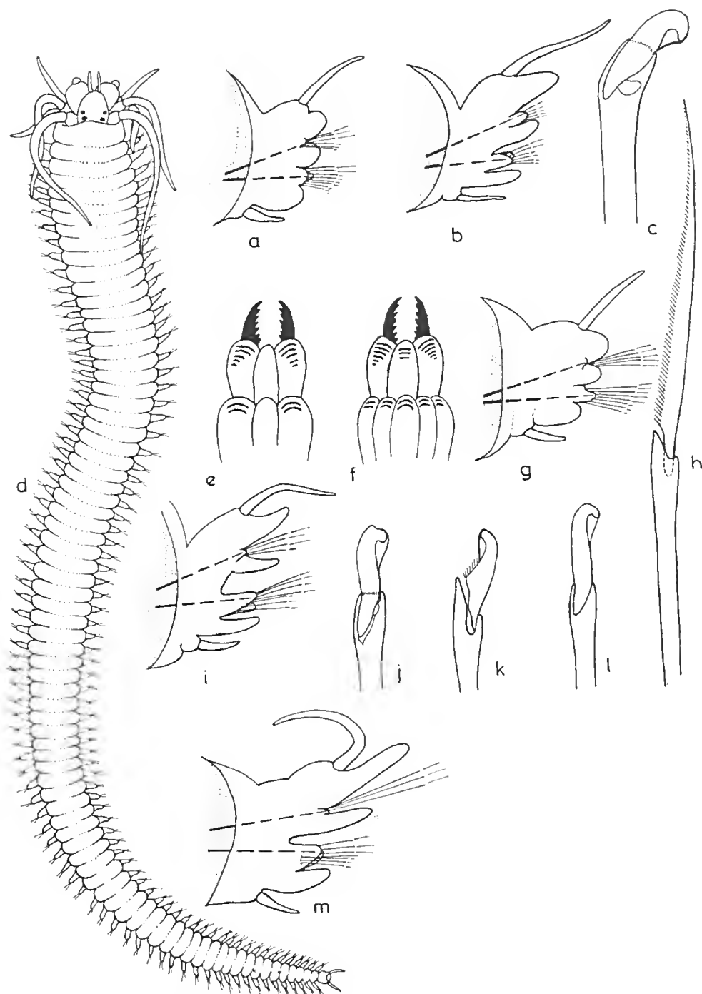
FIG. 14.4. Platynereis calodonta . (A) Anterior foot. (B) Posterior foot. (C) Homogomph falcigers. Platynereis dumerillii . (D) Entire worm. (E, F) Dorsal and ventral views of proboseis. (G) Anterior foot. (H) Heterogomph spiniger. (I) Posterior foot. (J) Notopodial falciger. (K) Neuropodial falciger. Platynereis isolita . (L) Notopodial falciger. Platynereis australis . (M) Posterior foot.
