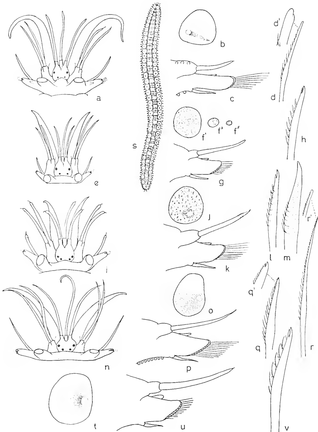
FIG. 1.16. Lepidasthenia mossambica . (A) Head. (B) Elytron. (C) Foot. (D) Neuroseta. Lepidasthenia microlepis . (E) Head. (F 1, 3, 5 ) First, third and fifth clytron. (G) Foot. (H) Neuroseta. Lepidasthenia elegans . (I) Head. (J) Elytron. (K) Anterior foot. (L) Normal neuroseta. (M) Giant neuroseta. Lepidasthenia brunnea . (N) Head. (O) Elytron. (P) Foot. (Q) Middle bidentate neuroseta. (R) Superior fine neuroseta. Lepidasthenia maculata . (S) Entire worm (natural size). (T) Elytron. (U) Foot. (V) Neuroseta.
