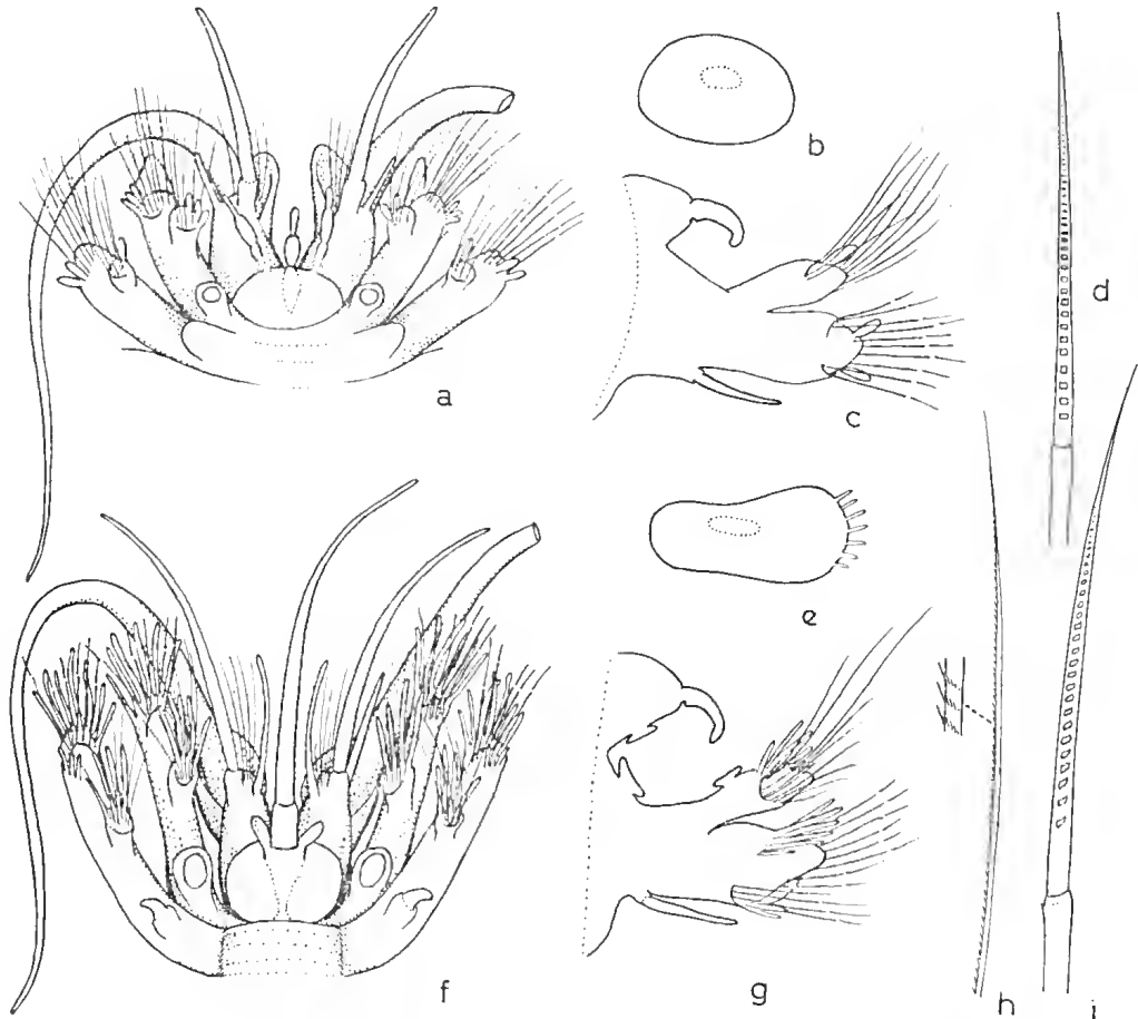
FIG. 1.21. Leanira hystrix . (A) Head. (B) Elytron. (C) Foot. (D) Neuroseta. Sthenolepis tetragona . (E) Elytron. (F) Head. (G) Foot. (H) Notoseta. (I) Neuroseta.
