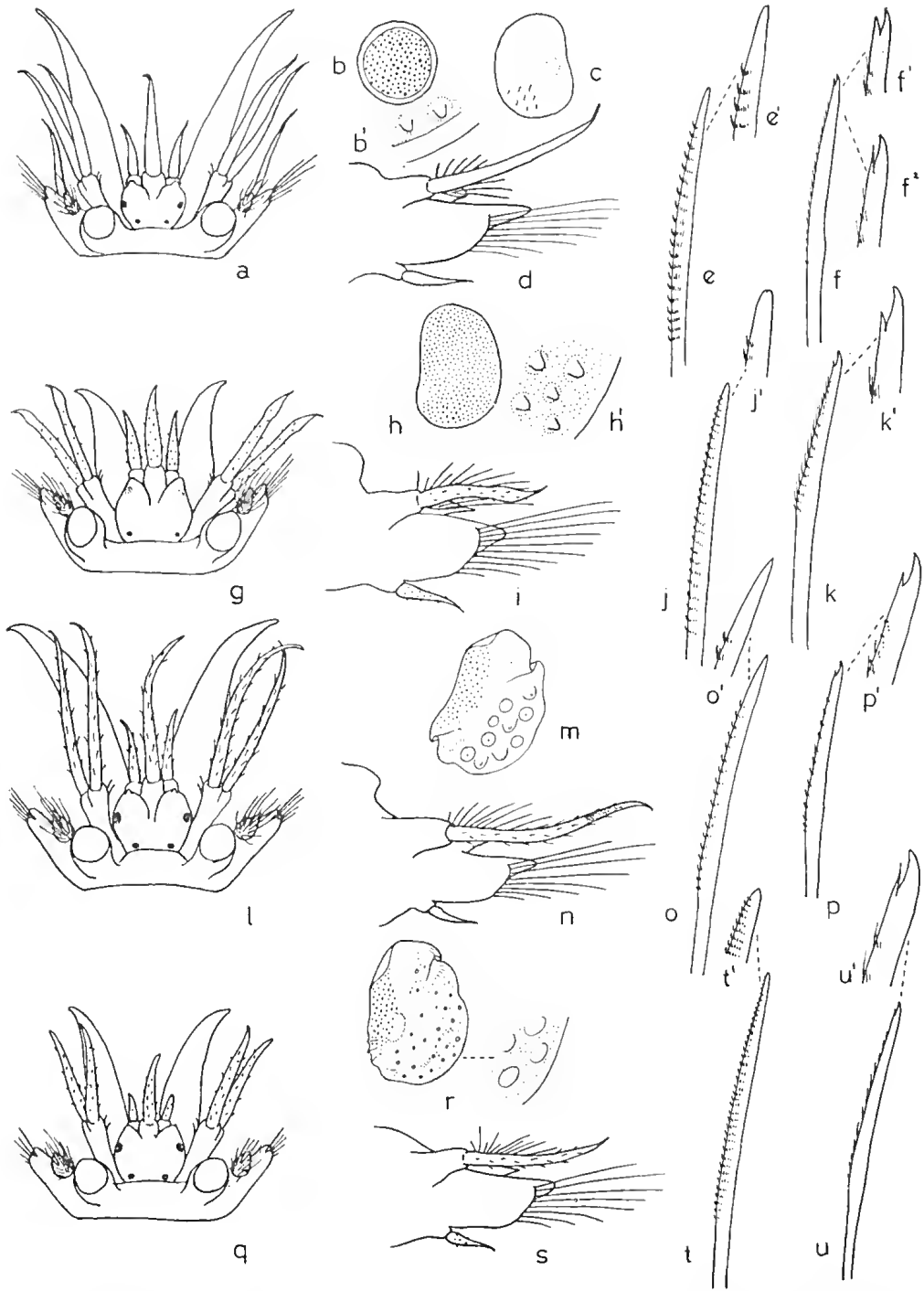
FIG. 1.11. Harmothoe corralophila . (A) Head. (B) First clytron. (C) Fifth clytron. (D) Foot. (E) Notoseta. (F) Neuroseta. Harmothoe waahli . (G) Head. (H) Elytron. (I) Foot. (J) Notoseta. (K) Neuroseta. Harmothoe fraserthomsoni . (L) Head. (M) Elytron. (N) Foot. (O) Notoseta. (P) Neuroseta. Harmothoe agulhana . (Q) Head. (R) Elytron. (S) Foot. (T) Notoseta. (U) Neuroseta.
