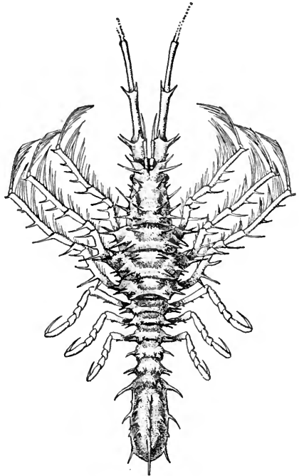
FIG. 366.—ARCTURUS FLORIDANUS.
