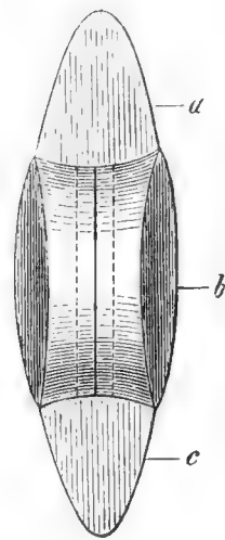
Fig. 2. Seitenansicht eines Haifschwirbels.
