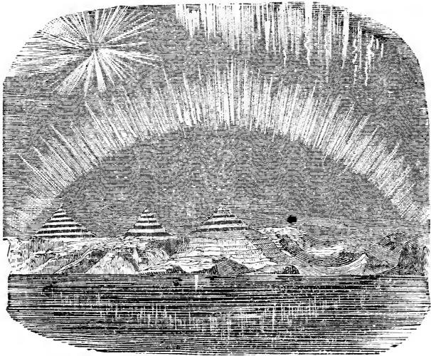
AURORA BOREALIS.
