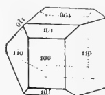
FIG. 2. Lævo-tartaric acid.
