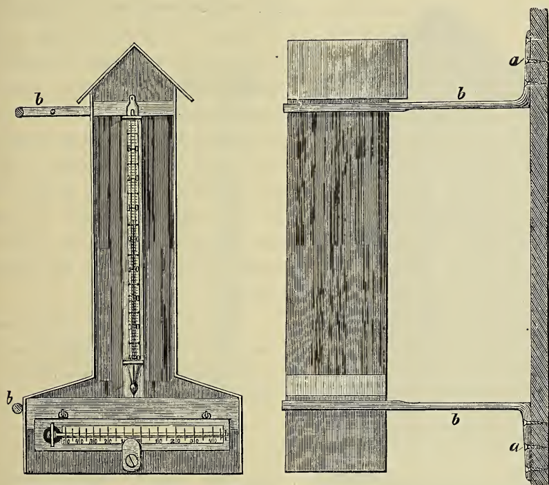
Fig. 27 og 28. Termometerhuse.
