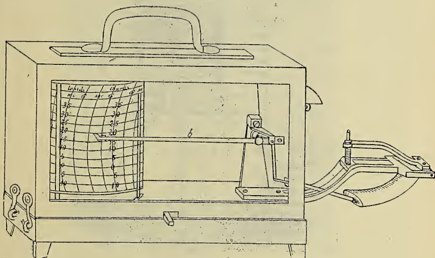
Fig. 24. Richards termograf.
