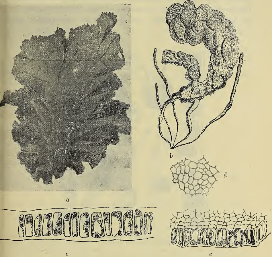
Fig. 40. Ulvacèer. a. Monostroma. b. Enteromorpha. c. Tversnit af løvet hos en ulvacè. d. Et stykke af løvet hos en ulvacè seet fra fladen. e. Schematisk fremstilling af løvets bygning hos en ulvacè.
