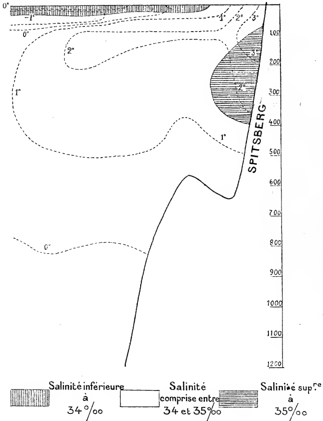
Fig. 6. Snit gjennem Golfstrømmen paa høiden av Spitsbergen. — Vand av saltholdighet under 34 pro mille er betegnet ved lodret, vand av saltholdighet over 35 pro mille ved vandret skræfning. Vand av saltholdighet mellem 34 og 35 pro mille er betegnet uten skræfning.
