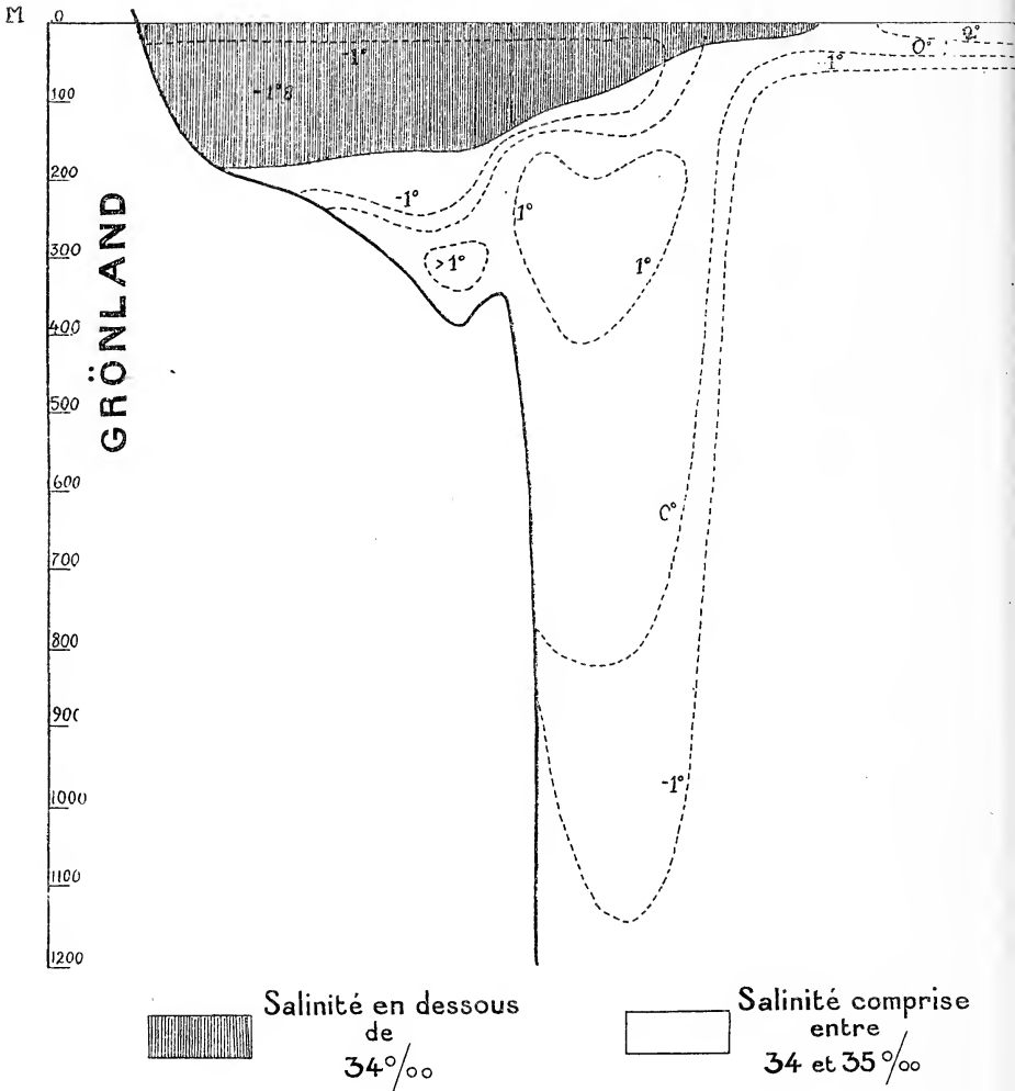
Fig. 4. Snit gennem Polarstrømmen utenfor Grønlands østkyst. — Vand med saltholdighet under 34 pro mille er betegnet ved lodret skraffering; vand av saltholdighet mellem 34 og 35 pro mille er betegnet uten skraffering.
