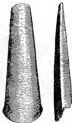
Fig. 2. Hyolithes. (Efter Kayser).
