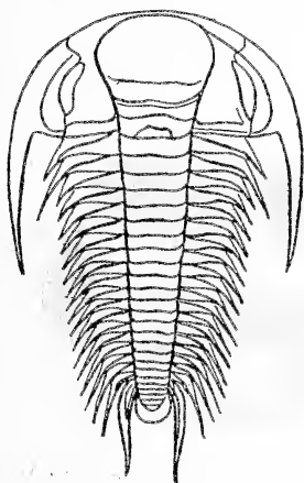
Fig. 1. Kambrisk trilobit. (Efter J. Walther).
