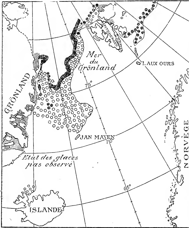
Fig. 2. Isforholdene i Grønlandshavet i juli 1905. — Den tykke sorte strek betegner grænsen for den sammenhengende polaris; landisens omraade er betegnet ved skraa skraffering, den tætte polaris ved sorte og den aapnere ved lyse cirkler.
