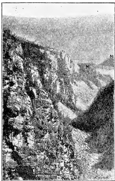
Fig. 4. Utsigt gjennom Jutulhugget mot Tyldalen. (M. er morænen).
