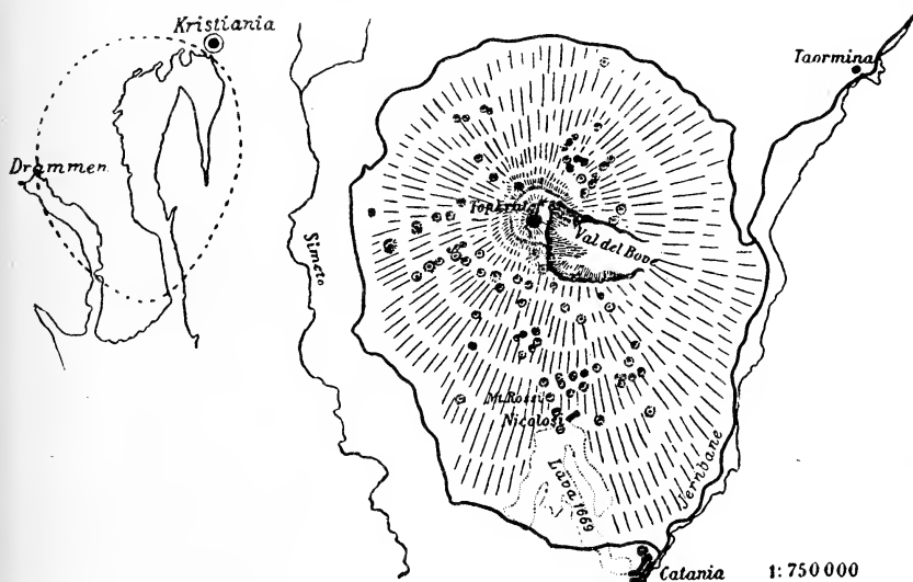
Fig 1. Etna. Tilvenstre Etnas grundflate (omskrevet med en punktert linje) sammenlignet med Kristianiafjordens omgivelser.
