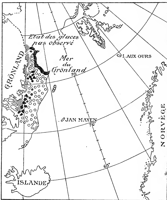
Fig. 3. Isforholdene i Grønlandshavet i august 1905. — De uregelmæssige sorte flekker betegner utstrakte ismarker. Kfr. forøvrigt figurforklaringen til fig. 2.
