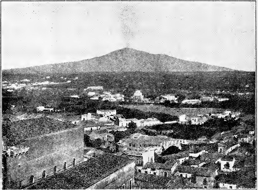
Fig. 2. Etna seet fra Catania, februar 1891.
