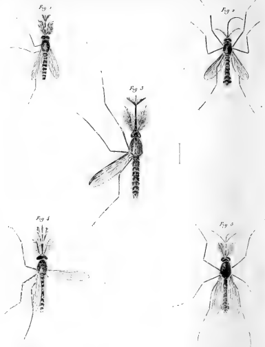
Fig. 1 Culex laticornis n. sp. Fig. 2 Culex (= Megarthria ) subulifer n. sp. Fig. 3 Culex (= Vere ) n. sp. Fig. 4 Culex subulifer n. sp. Fig. 5 Culex (= Megarthria ) ambrosensis n. sp.
