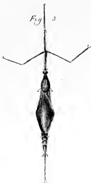
Fig. 1. Cylindrotoma albitarsis n. sp. Fig. 2. Sciophilala tropica n. sp. Fig. 3. Limnophila cruce n. sp.
