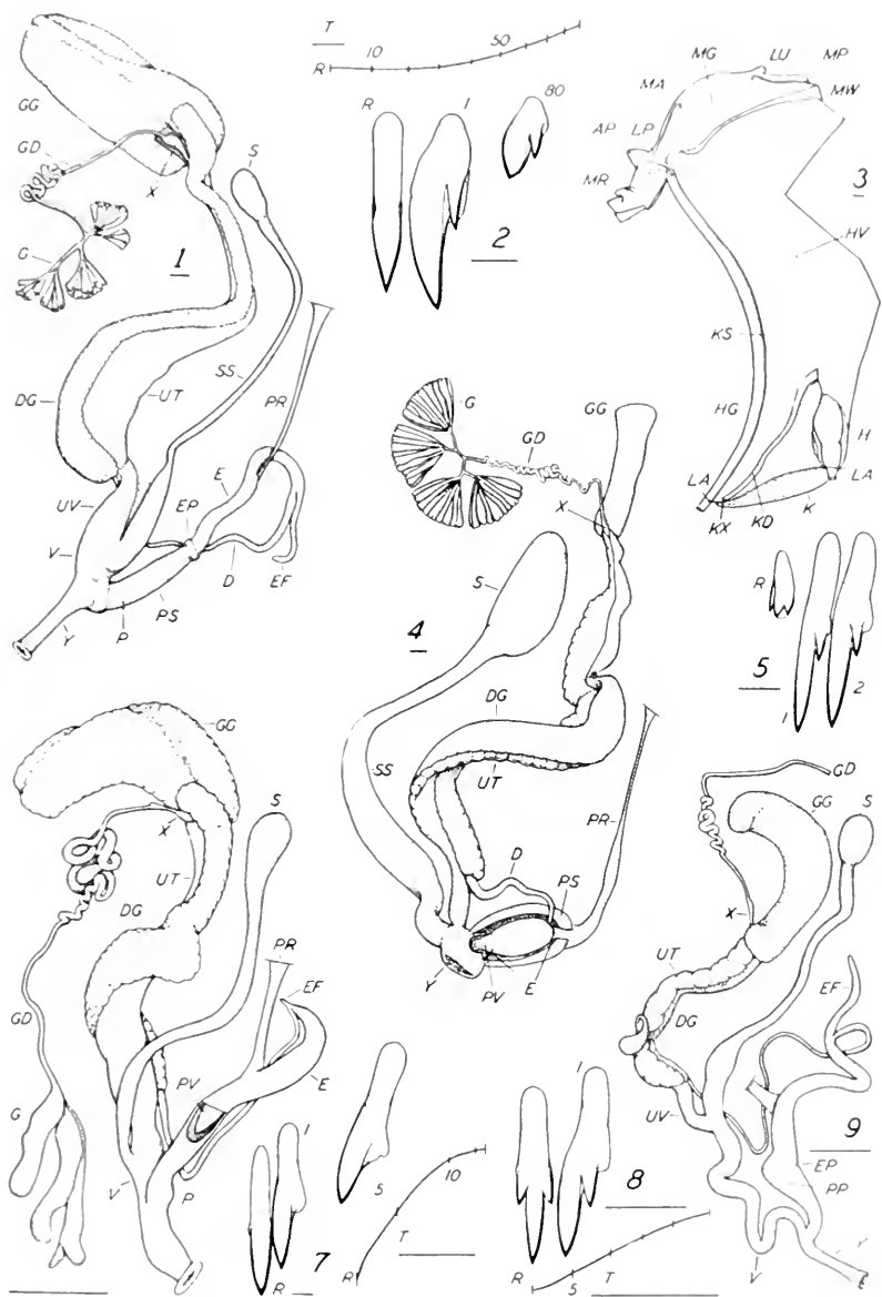
Figs. 1-3, Farulla buccinatus struthella . Fig. 4, Lacuna (P.) dubia . Fig. 5, F. provara . Figs. 6-7, Sigmatarias laevisculos . Figs. 8-9, F. acuta horrida .
