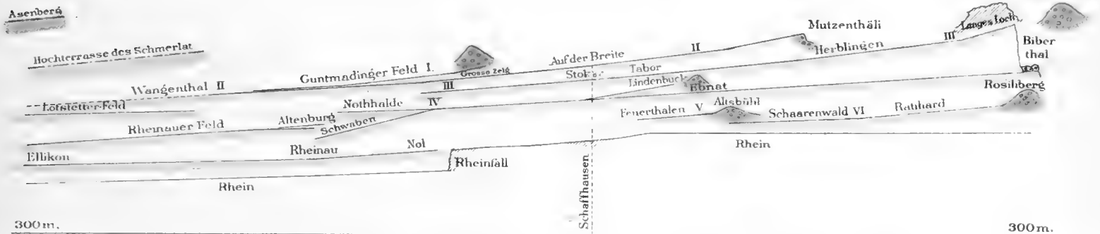
Längsprofil der Schaffhauser Terrassen. Längen: 1:100,000. Höhen: 1:5,000.
