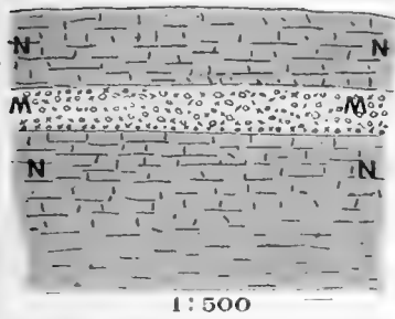
Profil im Steinbruch am Hohenegg. Stammheimer Berg. Moräne (M) in löcheriger Nagelfluh (N).
