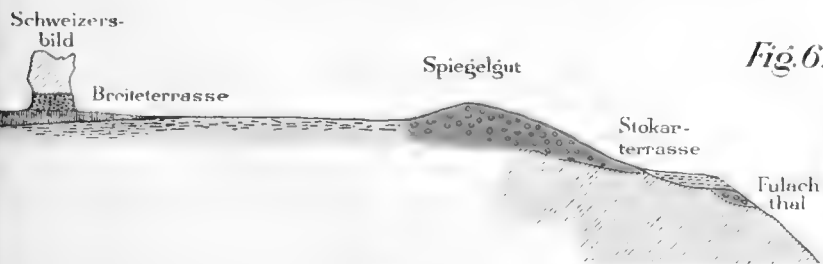
Profil vom Schweizersbild zum Fulachthal. Höhen 1:1250, Längen: 1:12,500.
