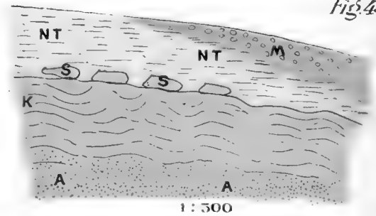
Profil der Kalktuffgrube von Flurlingen. Moräne (M) über Glazialschotter (NT) an der Basis mit grossen Kalktuffschollen (S) Darunter fester Kalktuff (K) unterteuft von lockerem (A).
