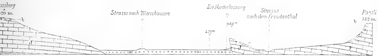
Fig. 2. Schnitt durch das Schweizersbildthal.
