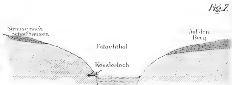
Querprofil durch das Fulachthal am Kesslerloch. Höhen und Längen 1:1250.
