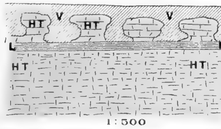
Profil in der Schottergrube am Schmerlat. Loser Hochterrassenschotter (HT) überlagert von einem Mergelbande (L) im Hangenden des- selben zu Nagelfluh verkitet. (HT) von weicher pilzförmige Partien in den Verwitterungslehm (V) hineinragen.
