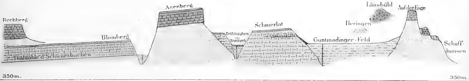
Längsprofil durch das Klettgau. Längen: 1:100,000 Höhen: 1:5,000.
