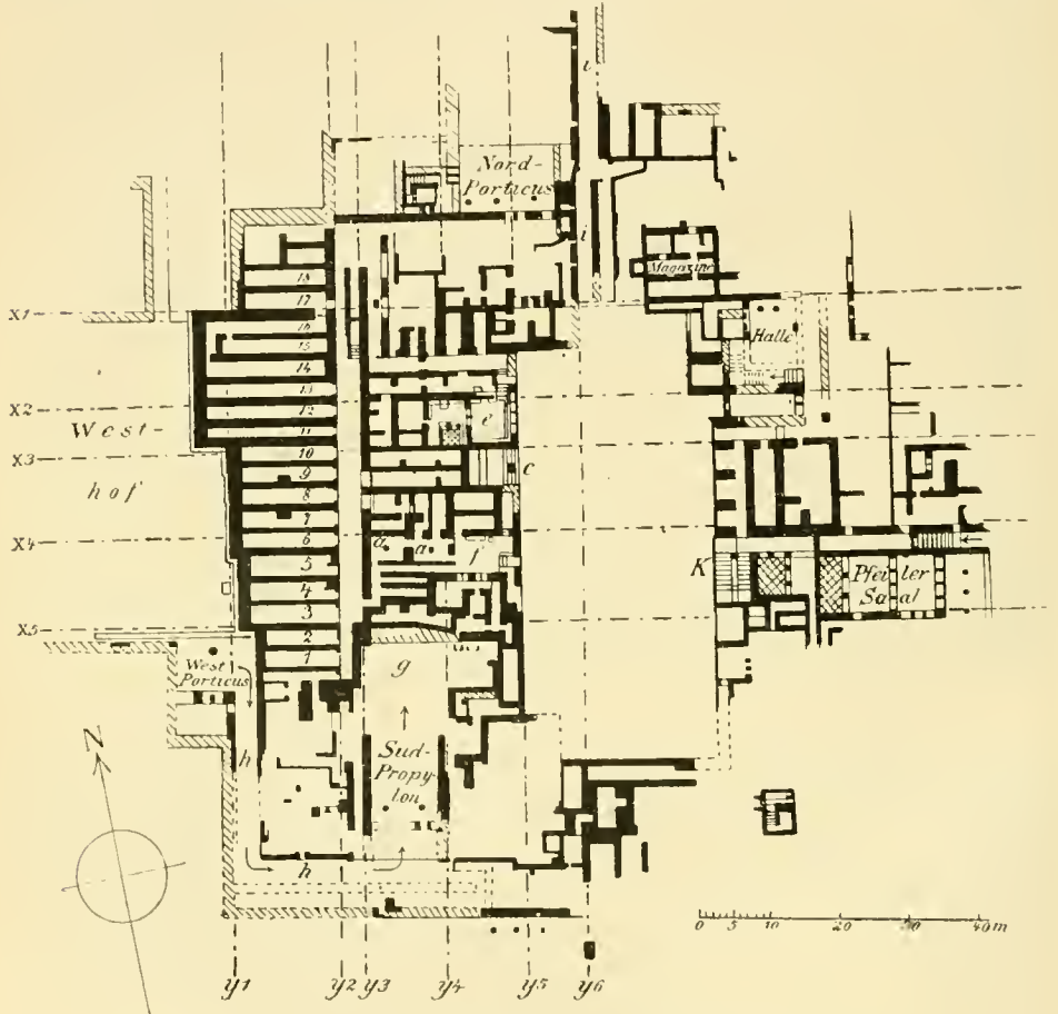
2. Grundriß des Palastes zu Knosos (1901)
