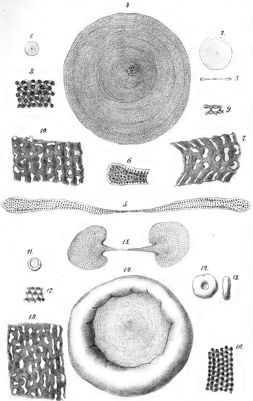
1-10 Orbitolites praecursor G ü m b .
