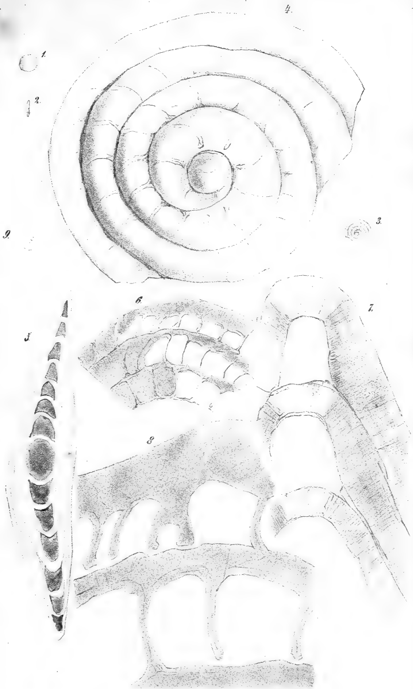
1-8 Nummulites jurasica Gümb.
