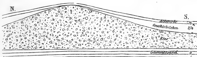
Fig. 1. Profil in der Kiesgrube bei Seifersdorf.
