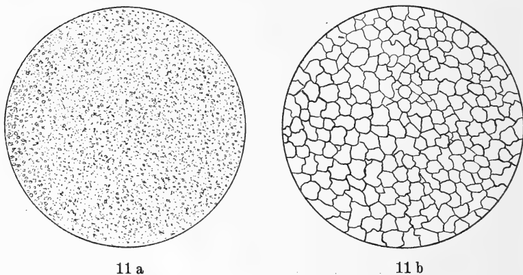
Fig. 11. a) Solenhofener Kalkstein. b) Durch Sammelkristallisation im festen Zustande zusammengeflossene Kalkspatteile des Solenhofener Kalksteins (Marmorisierung).
