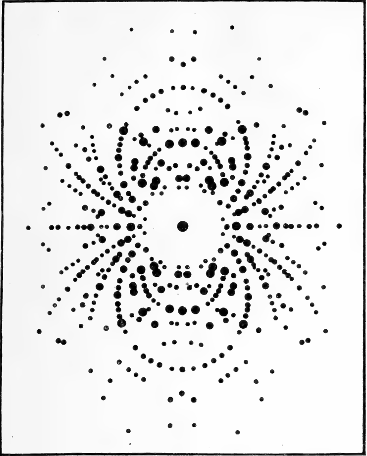
Fig. 22. Lauediagramm von Olivin auf {001}.
