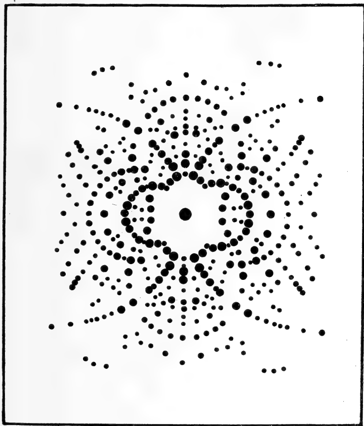
Fig. 29 b. Lauediagramm von Aragonit auf {010}.
