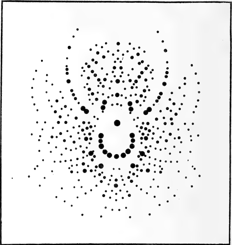
Fig. 26 a. Lauediagramm von Sanidin auf {001}.
