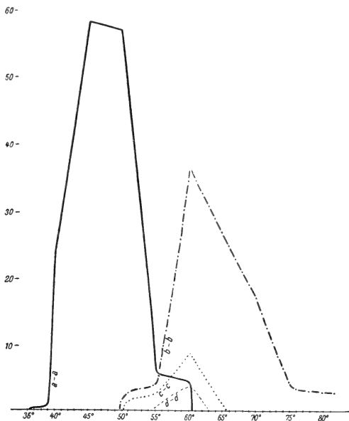
Fig. 17. Derselbe Linienvorlauf für das gleiche Material nach seiner Trennung und Verteilung auf die verschiedenen stratigraphischen Stufen.
