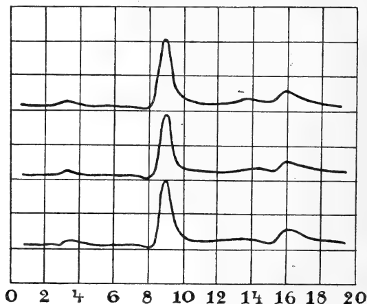
Fig. 10. Übereinstimmende Reflexmaxima bei den wasserhaltigen Sulfaten von Mg-K, Co-K, Zn-K. Nach CL. SCHAEFER und M. SCHUBERT. Zahlen geben \lambda in \mu .
