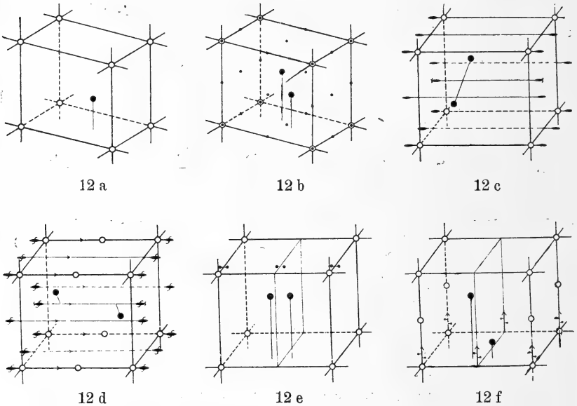
Fig. 12. Die sechs grundlegenden kristallstrukturellen Schemata.
