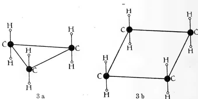
Fig. 3 a, b. Moleküle von Trimethylen und Tetramethylen.
