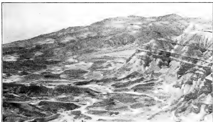
Fig. 3. Im Vordergrund rechts: Basalt, dem Miocän konkordant eingelagert. Im Hintergrunde Höhen aus Nummulitenkalk. Wadi Tayiba, westlicher Sinai.
