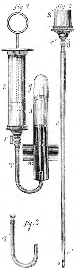
Fig. 77. — Appareil pour recueillir du sang Fig. 78. — Appareil gradué pour les analyses à l'abri du contact de l'air (Cl. Bernard) (*). de gaz du sang (Cl. Bernard) (**).
