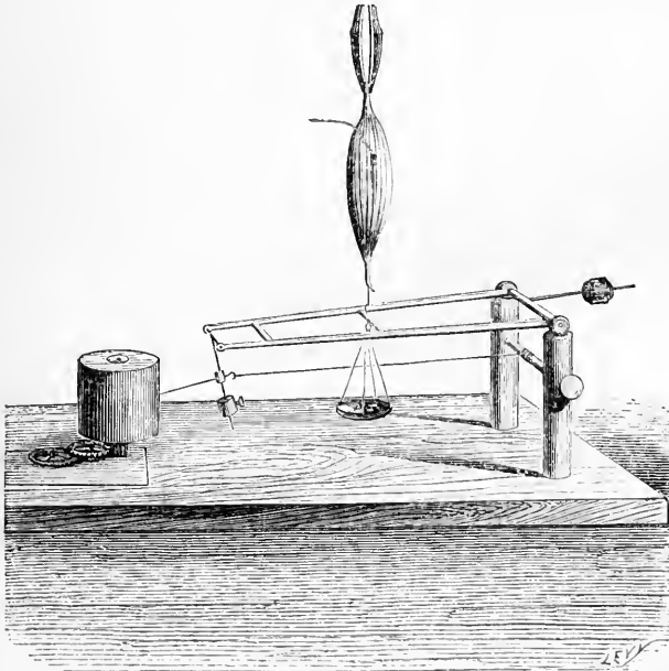
Fig. 127. — Myographe d'Helmholtz.
