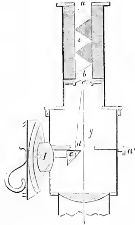
Fig. 73. — Microspectroscope oculaire.
