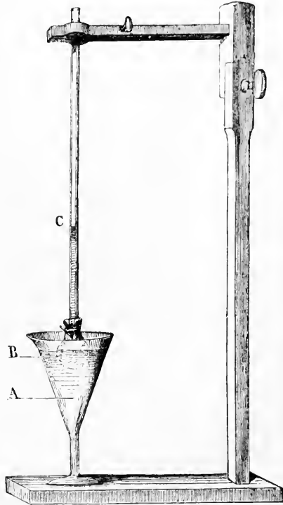
Fig. 100. — Endosmomètre.
