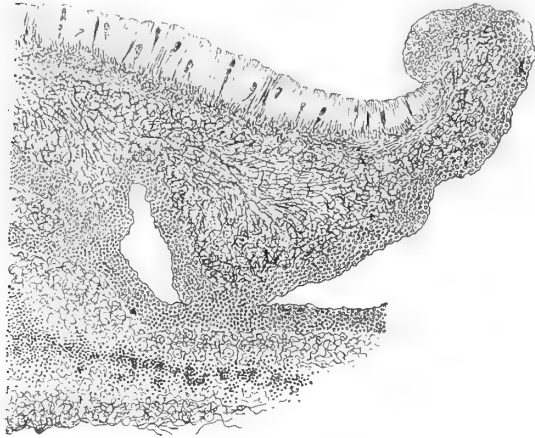
Fig. 12. — Pannaria lurida (Mont.) Nyl.
