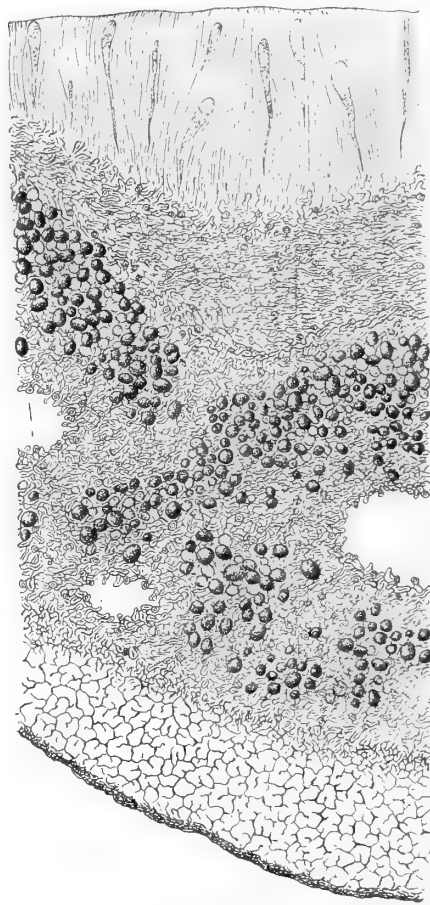
Fig. 6. — Lecanora subfusca var. allophona Ach.
