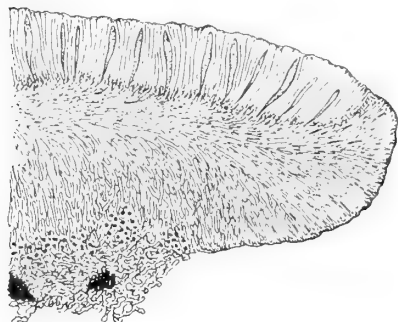
Fig. 10. — Lecideum rosella Ach.
