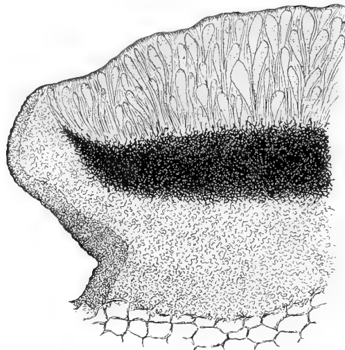
Fig. 14. — Lecanora mesoxantha Nyl.
