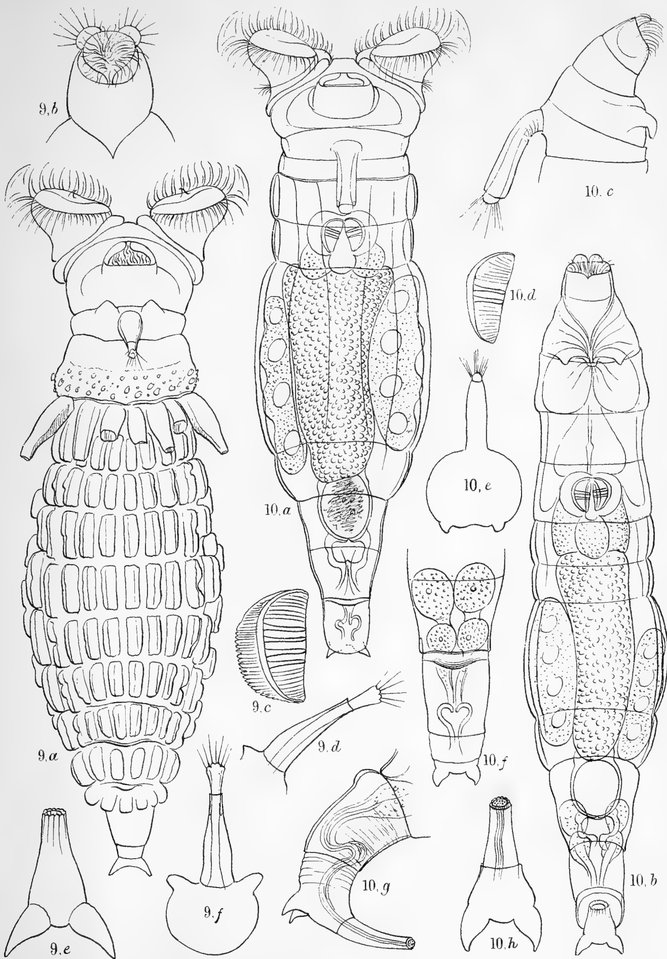
9, CALLIDINA INCRASSATA, n. sp.
