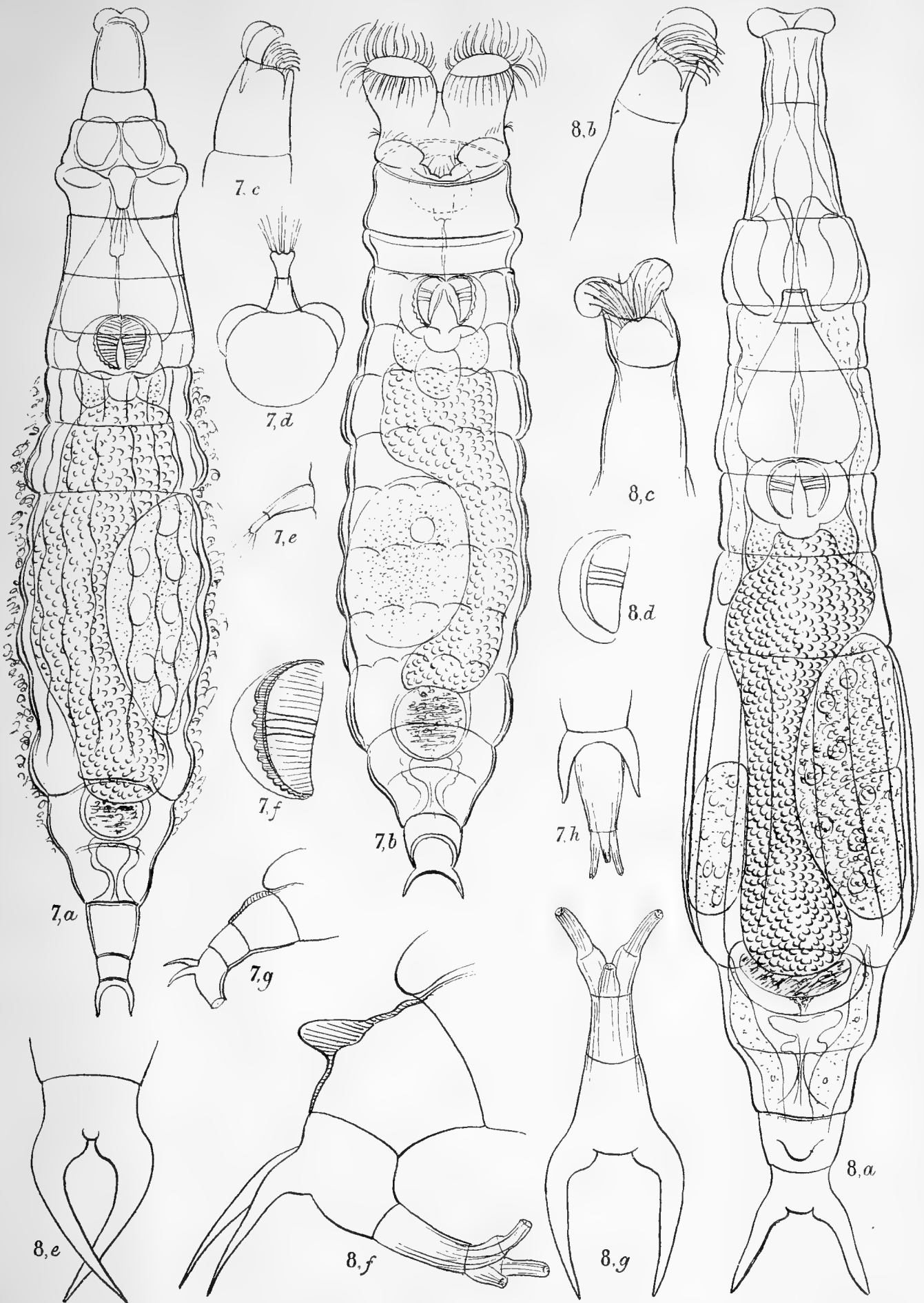
7, CALLIDINA MURICATA , n. sp.
