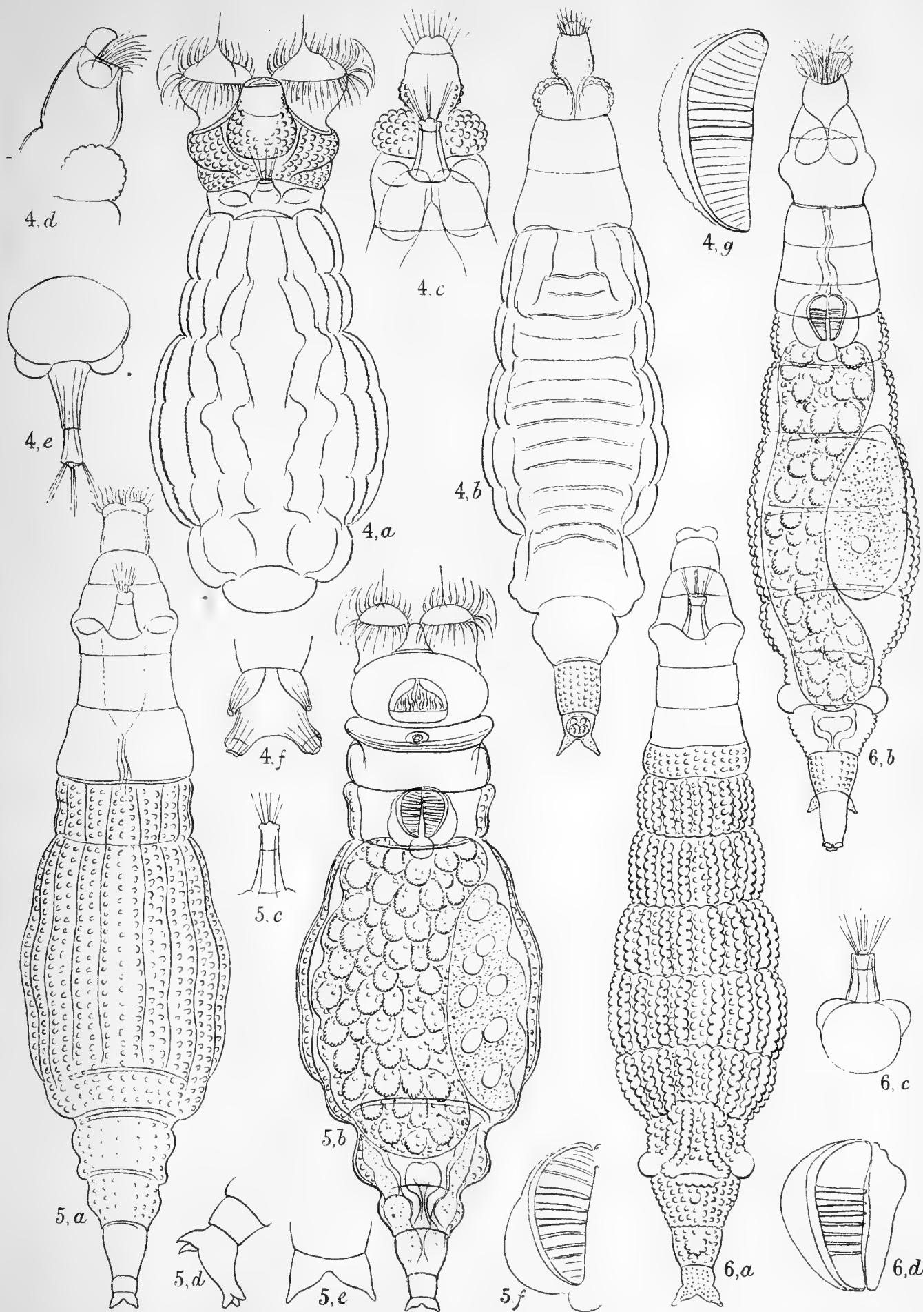
4, PHILODINA HUMEROSA, n. sp.
