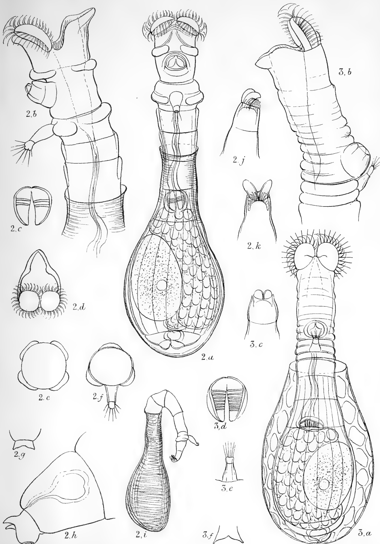
3, CALLIDINA ANNULATA, n. sp.
