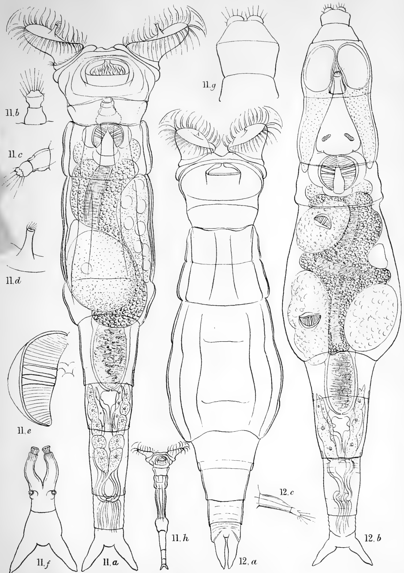
11, PHILODINA LATICEPS, n. sp.
