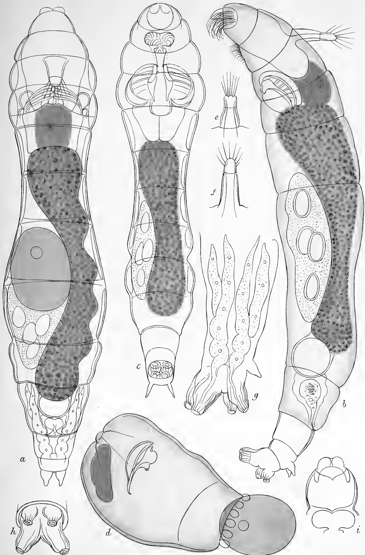
MICRODINA PARADOXA, n. sp.
