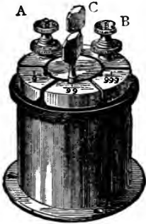
FIG. 158.—The Shunt.
