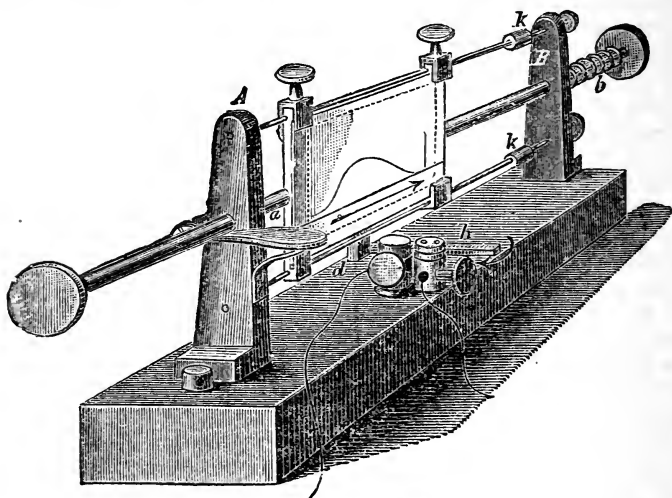
FIG. 127.—Spring-Myograph.
