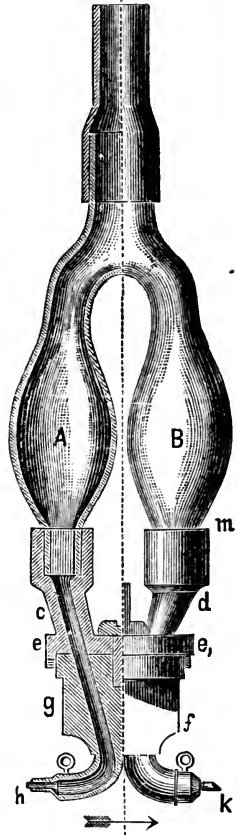
FIG. 222.—Rheometer.
