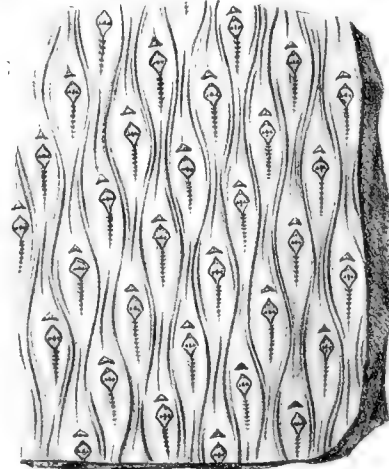
1. Lepidodendron rimosum Sternbg. — 2. Lepidod. crenatum Sternbg. — 3. Lepidod. Veltheimianum Sternbg. — 4. Lepidod. dilatatum Lindl. et Hufl. — 5. Stigmeteria frondis Brong. — 6. Lepidod. rimosum Sternbg. — 7. Lepidod. caudatum Sternbg. — 8a. Lepidod. Sternbergi Lindl. et Hufl. b. Lepidod. obovatum Sternbg. — 9. Stipillaria elegans Brong. — 10. Lepidostichus carabalis Lindl. et Hufl.
