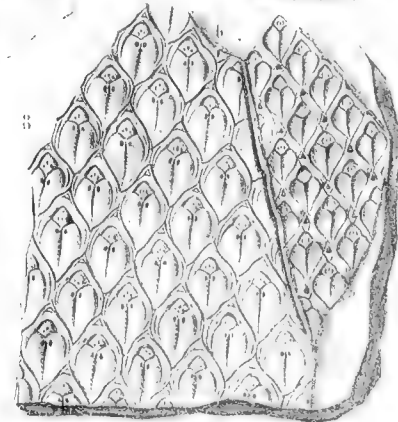
1. Lepidodendron rimosum Sternbg. — 2. Lepidod. crenatum Sternbg. — 3. Lepidod. Veltheimianum Sternbg. — 4. Lepidod. dilatatum Lindl. et Hufl. — 5. Stigmeteria frondis Brong. — 6. Lepidod. rimosum Sternbg. — 7. Lepidod. caudatum Sternbg. — 8a. Lepidod. Sternbergi Lindl. et Hufl. b. Lepidod. obovatum Sternbg. — 9. Stipillaria elegans Brong. — 10. Lepidostichus carabalis Lindl. et Hufl.
