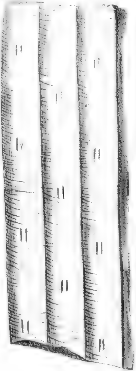
1. Sigillaria ocellata Sternbg. — 2. Sigillaria tessellata Bronq. — 3. Sigillaria Baumberti Roehl. — 4. Sigillaria mamillaris Bronq. — 5. Sigillaria intermedia Bronq. — 6. Sigillaria Boblayi Bronq. — 7. Sigillaria minima Bronq. — 8. Sigillaria pes-capraei Goldenb.
