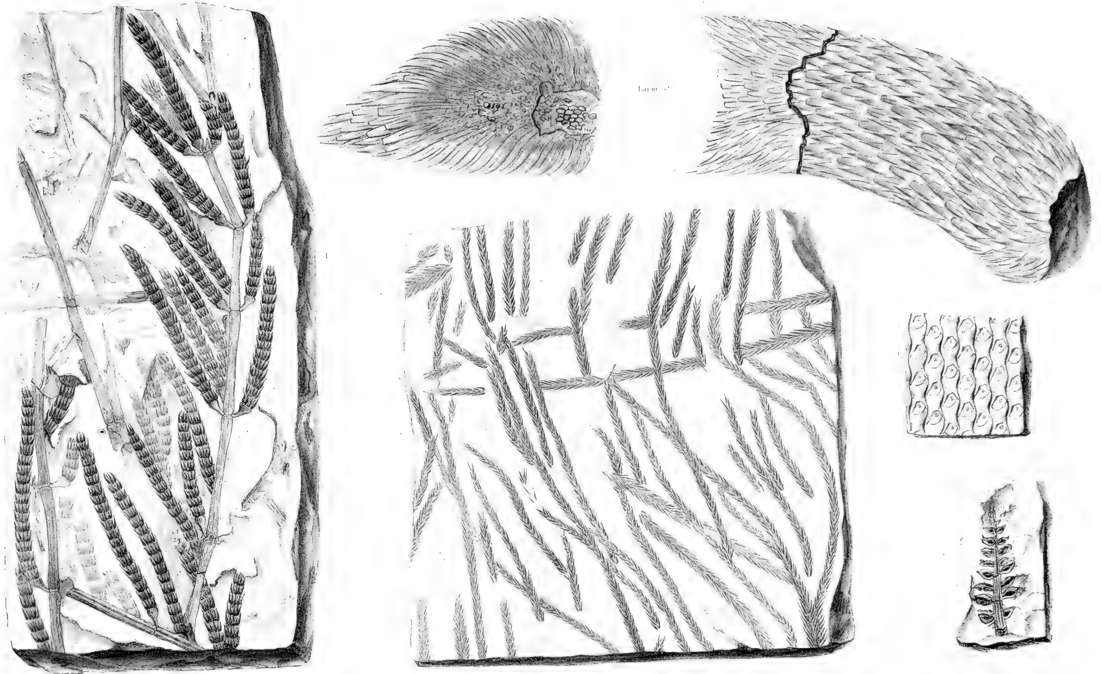
1. Volknamia elongata Presl. 2. Lepidostrobus variabilis Lindl et Hutt. 3. Lycopodites selaginoides Sternbg. 4. Sigillaria Dournasi Brongn. 5. Antholithes Pitarnuae Lindl et Hutt var. distans Andra
