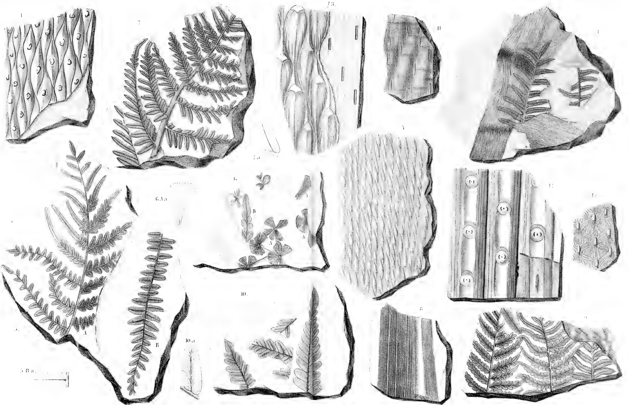
1. Lepidodendron undulatum Sternbg. 2. 5. 9. Aethopteris heterophylla Goepf. 3. Stigmaria conferta Corda. 4. Noeggerathia Benettiana Goepf. mit Aethopteris lonchitides Sternbg. 6. A. Sphenophyllum emarginatum Bry. 7. Bronnaria tenuis Coen et Schindler. 8. Odontopteris oblongifolia Roemer. 9. Lepidodendron polyphyllum Roemer. 10. Noeggerathia palmariformis Goepf. 10. Odontopteris neuropteroides Roemer. 11. Sigillaria muralis Roemer. 12. Sigillaria Lanzii Benning Roemer. 13. Lepidodendron barbata Roemer.
