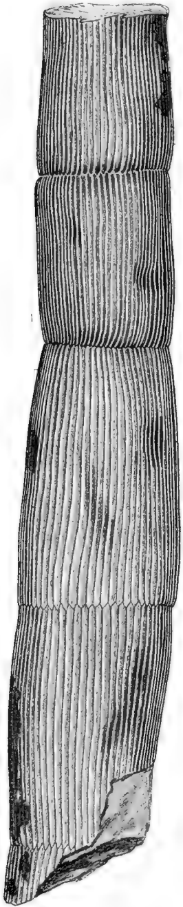
1 Calamites canaliculatus Schloth 2 Calamites Suckowii Brong 3 Calamites canaliculatus Schloth 4 Lepidostrobilus variabilis C. Lindl et Hutt 5 a Pinnularia capillaris Lindl et Hutt b B. n. hist von Lepidophellon mapis Brong 6 Asterophyllites (Leatulus) ... 7 Calamites approximatus Schloth
