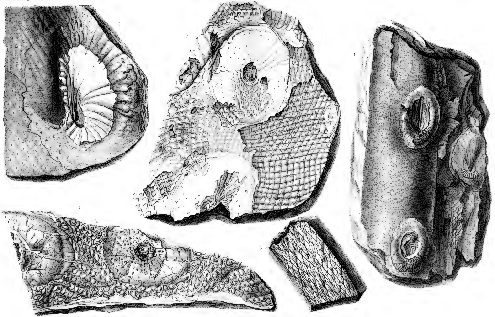
1. Clodendron Lindleyanum Sternbg. 3. Clodendron ellipticum Sternbg. 5. Lepidodendron Veltheimianum Sternbg.
