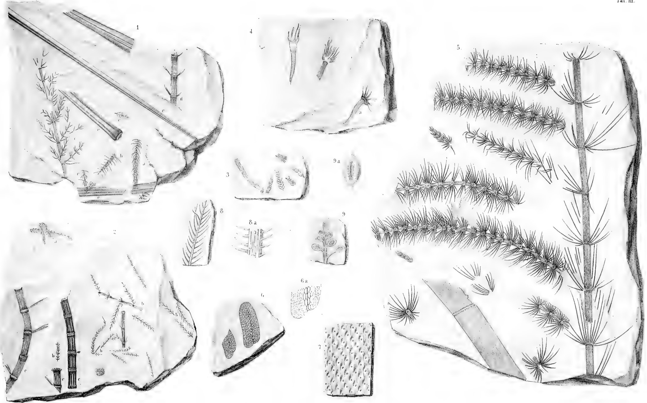
1a b c Asterophyllites delicatula Brong, d Sphenophyllites spec, e Sigillariae foliae. 2, a b Asterophyllites delicatula Brong, c Sphenophyllites saxifragae-folium Sternb. 3 Asterophyllites delicatula Brong 4 Asterophyllites spec 5 Asterophyllites equisetiformis Schloth 6 Dictyopterus obliqua Bumburg. 7 Lepidodendron Suckowiana Geinitz. 8 Asterophyllites fenella F. A. Roemer. 9 Carpolites distichus F. A. Roemer
