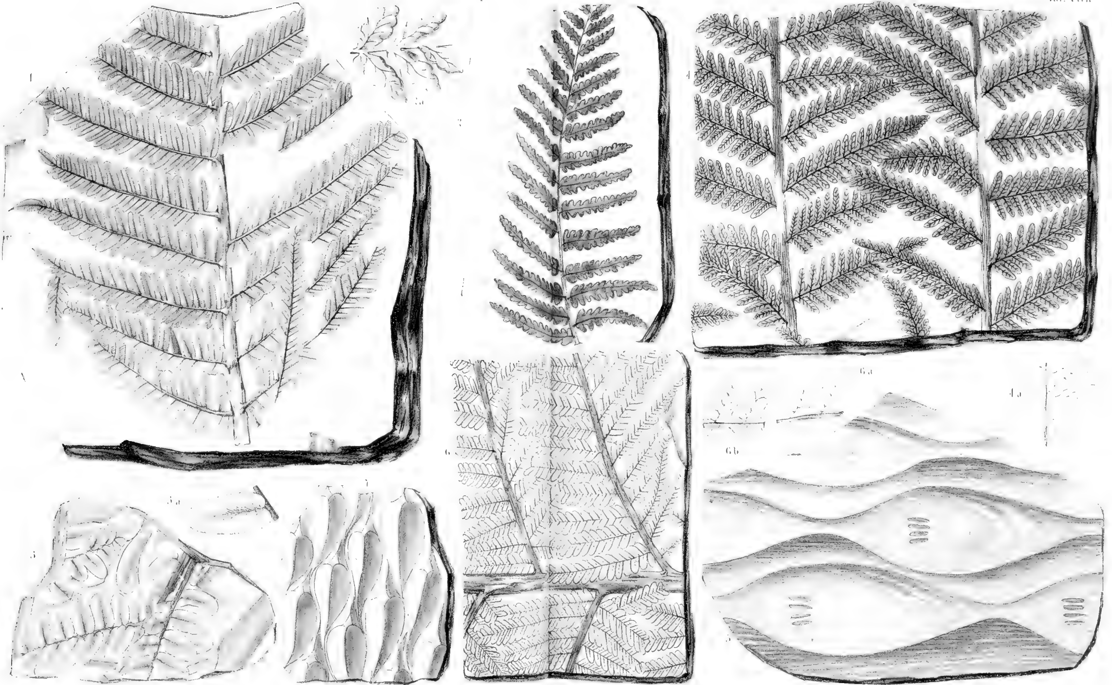
1. Xenopteris ovata Hoffmann. 2. Sphenopteris Pagenstecheri F. A. Roemer. 3. Xenopteris heterophylla Sternbq. 4. Peropteris plumosa Brong. 5. Caulopteris macrodiscus Sternbq. 6. Cyatites dentatus Goepf. 7. Lepidodendron Pagenstecheri F. A. Roemer.
