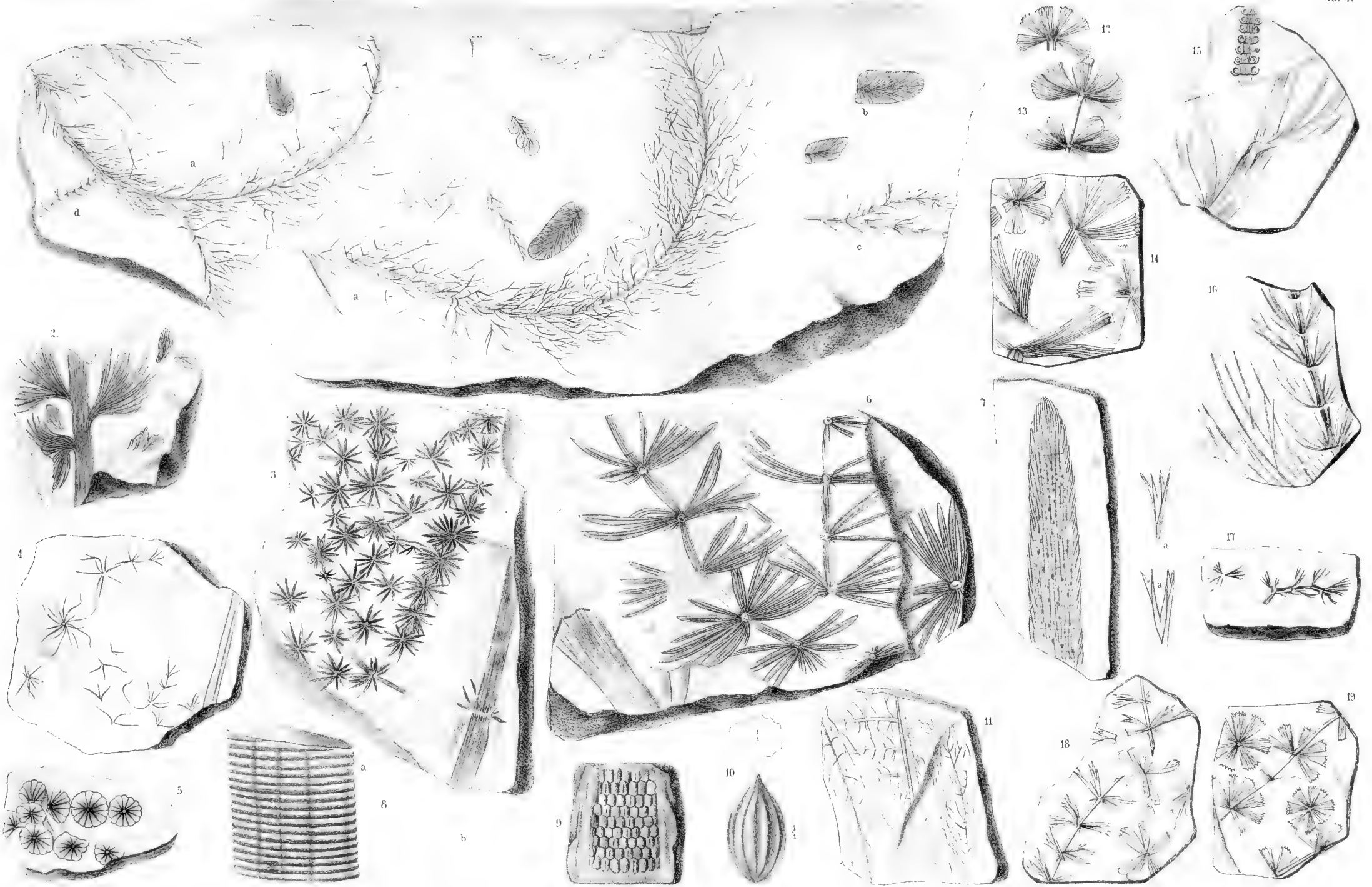
1a. Annularia capillacea Lindl. et Hutt., b. Fiederchen von Neuropteris flexuosa Sternbg., c. d. Asterophyllites delicatula Brq. 2. Odontopteris Reichiana v. Gutb. 3. 4. Annularia radiata Sternbg. 5. Annularia sphenophylloides Zenk. 6. 15. Annularia longifolia Brq. 7. Vollmannia major Germ. 8. Artisia transversa Presl. 9. Equisetites infundibuliformis Bronn. 10. Trigonocarpon ellipsoideum Goepf. 11. Sphenophyllum Schlotheimii Brq. 12. Sphenophyllum emarginatum Brq. 13. Sphenophyllum longifolium Germ. 14. Sphenophyllum longifolium Germ. 16. Asterophyllites longifolia Sternbg. 11. Sphenophyllum saxifragae-folium Sternbg. 13. Sphenophyllum angustifolium Germ. 19. Sphenophyllum crossum Lindl. et Hutt.
