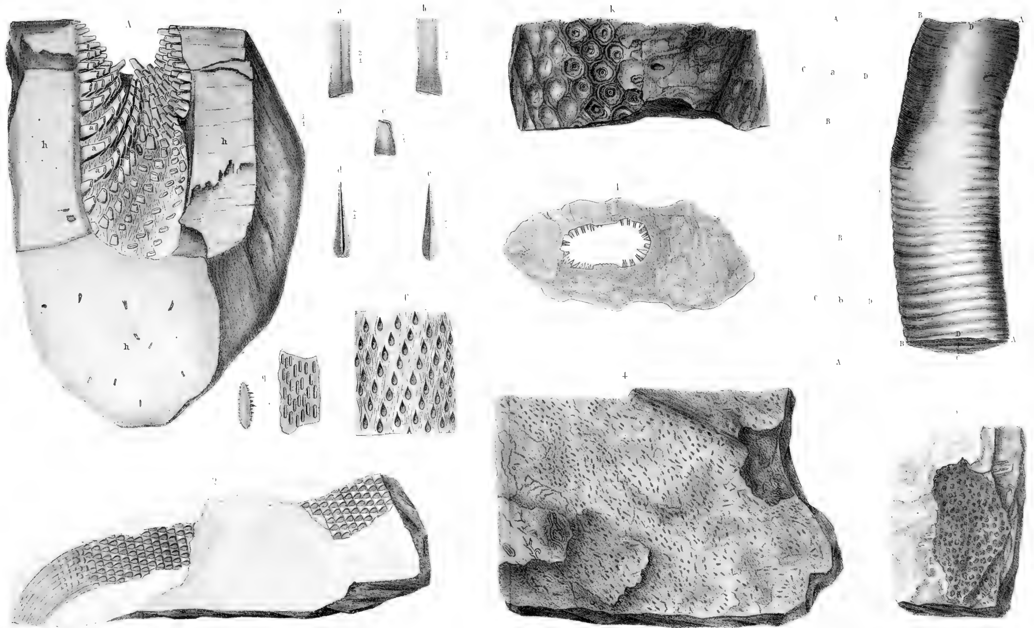
1. Stigmaria ficoides Brong., A Querschnitt eines Stammes mit der Höhlung des Holzzylinders, a, b, c, d, e, Markstrahlen f. füllte Percha Abdrücke der Höhlung, g Stück des Markkerns, h, ausgefüllte strukturlose Masse, k Stammstück mit Blattnarben auf der Oberfläche, l, Durchschnitt desselben — 2. Huttonia carinata Germ. — 3. Lomdophloyos crassicaule Corda ( Artisia approximata Enger.) — 4. 5. Selaginites Erdmanni Germ.
