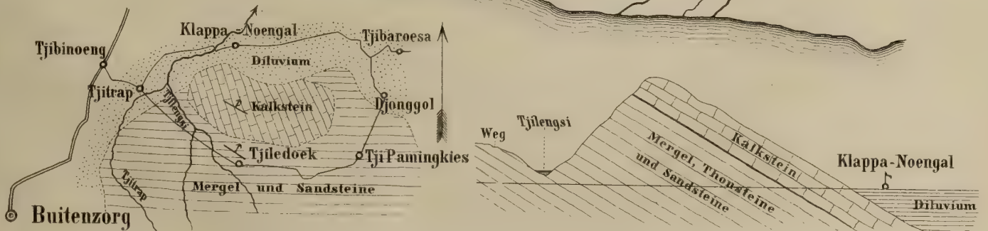
Fig. 3. Geologische Kartenskizze der Gegend östlich von Buitenzorg. Insel Java.
