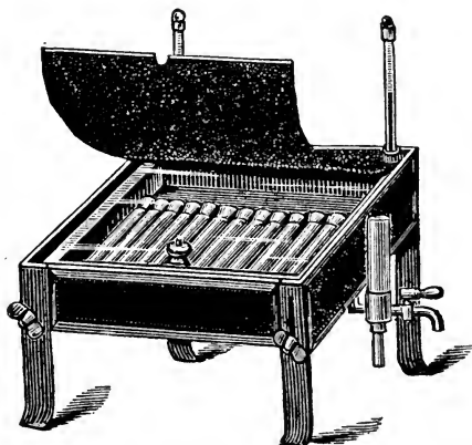
FIG. 35.—Koch's serum sterilizer.
