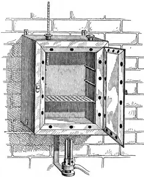
FIG. 28.—Hot-air sterilizer.
