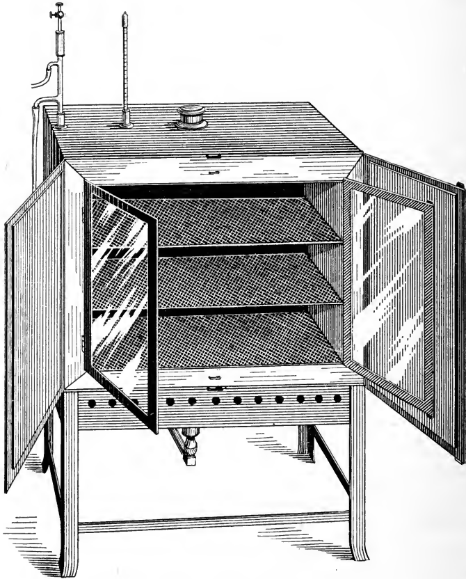
FIG. 46.—Incubator.
