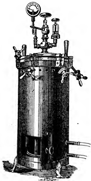
FIG. 32.—Autoclave.
