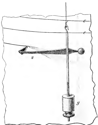
Fig. 9. s Schreibfeder; g Spangewicht. Ueber andere Constructionen der Schreibfeder vgl. z. B. Langendorff, l. c. p. 44.
