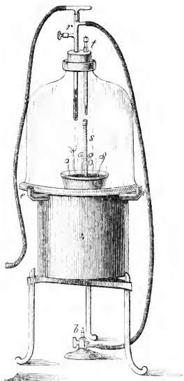
Fig. 17. Das Zinkgefäss z ist zwischen der doppelten Wandung mit Wasser gefüllt. Durch den Thermoregulator r wird die Flamme und somit die Temperatur des Glockenraumes regulirt. t und s Thermometer.
