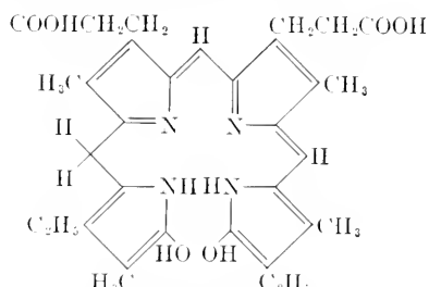
(II) Seidel's mesobilirhodin (= phycoerythrobilin?)
