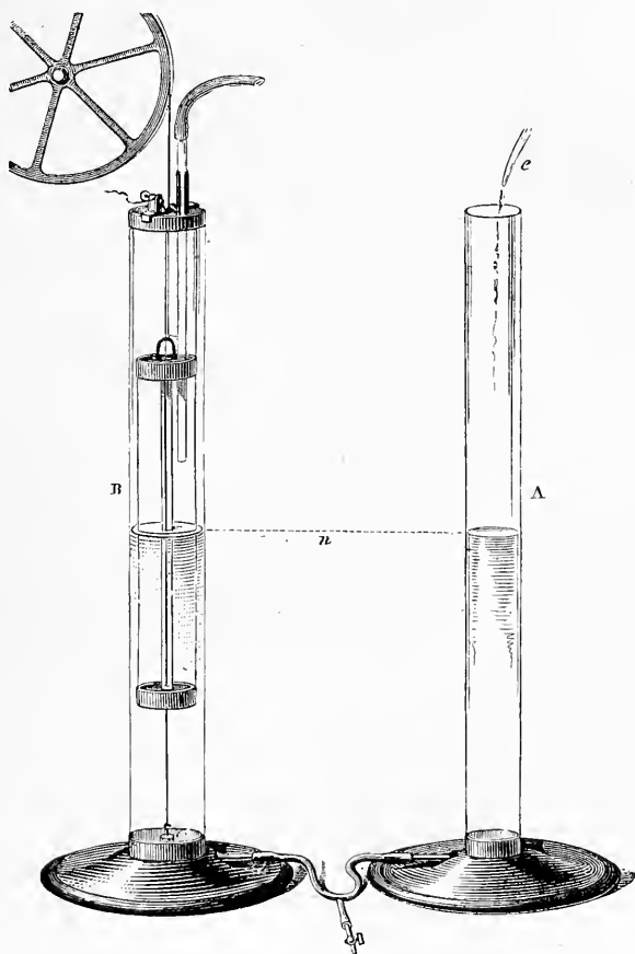
Fig. 86. — Flotteur inscrivant la courbe d'un écoulement de liquide. A et B vases communicants; e orifice d'écoulement; n niveau graduellement croissant de l'eau dans les deux vases. Du flotteur qui remplit presque entièrement le diamètre du vase B, se détache un fil qui passe sur une large poulie d'aluminium, et va actionner le style inscripteur représenté figure 87.
