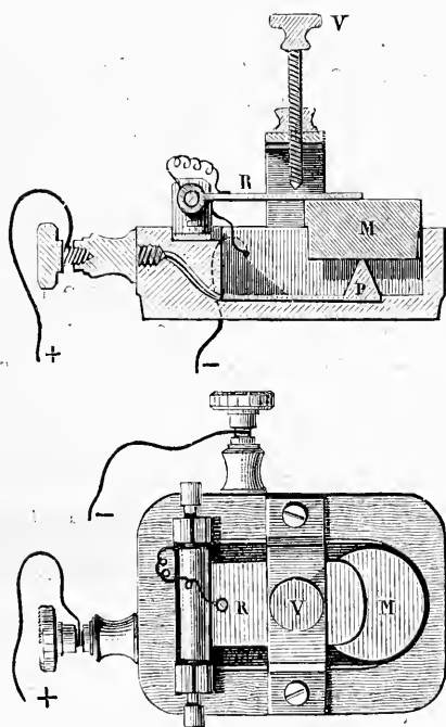
Fig. 61. — Explorateur électrique des vibrations du larynx (coupe et élévation).
