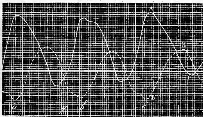
Fig. 83. Courbes des deux ordres de mouvement de l'aile d'un pigeon. — AP, ligne pleine, mouvements dans le sens antéro-postérieur. — HB, ligne ponctuée, mouvements de haut en bas.
