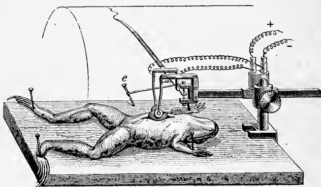
Fig. 24. — Myographe du cœur.
