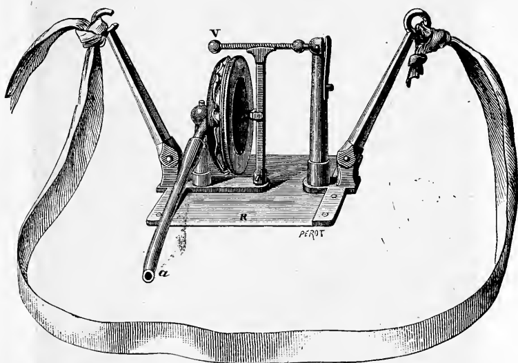
Fig. 77. — Pneumographe ou explorateur des mouvements respiratoires.
