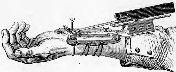
Fig. 102. — Sphygmographe direct en position sur le poignet.
