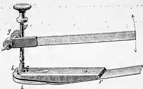
Fig. 101.—Disposition nouvelle du ressort et du levier du sphygmographe: i , plaque d'ivoire qui s'appuie sur l'artère avec une pression qui dépend de la tension du ressort r ; b , vis verticale qui, par un mouvement de bascule, s'applique contre un galet g avec lequel elle engrène, de manière à entraîner le levier inscripteur.
