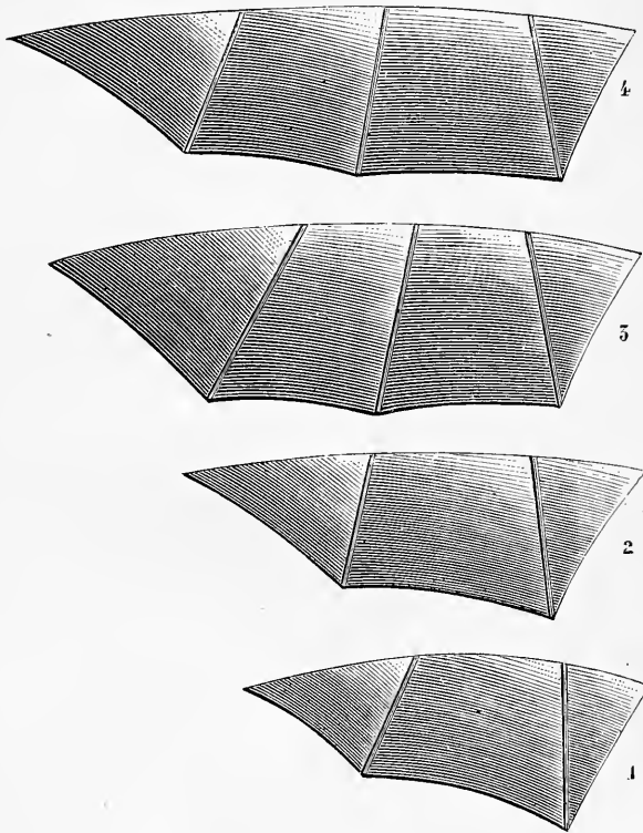
Fig. 37. — 1. Première paire d'ailes, représentant à peu près la voilure de la huppe. — 2. 2 e paire: la même un peu grandie. — 3. Ailes agrandies de beaucoup. — Ces 3 paires n'ont pas donné de résultats satisfaisants. — 4. Dernière paire, avec laquelle l'appareil vole très-bien.
