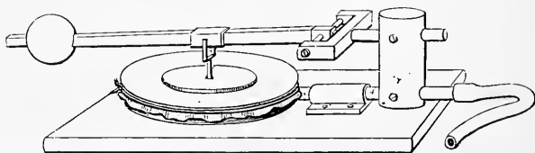
Fig. 79. — Tambour explorateur des oscillations. Cet appareil s'applique à l'étude des réactions verticales ou horizontales qui accompagnent les différentes allures de l'homme ou des animaux, à l'étude des oscillations du corps de l'oiseau pendant le vol, etc.
