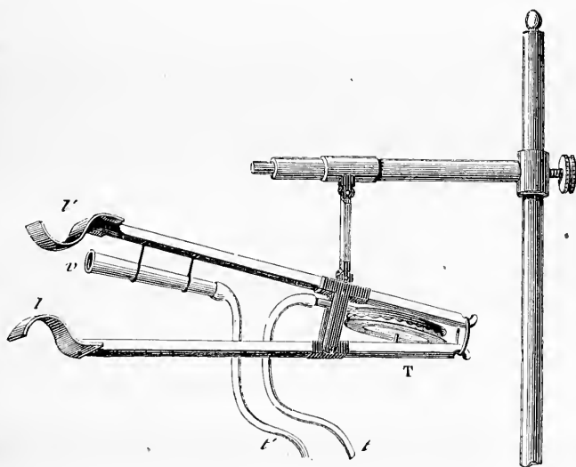
Fig. 63. — Appareil explorateur des mouvements verticaux des lèvres.
