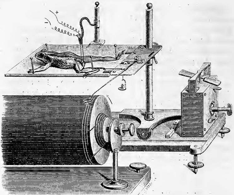
Fig. 68. — Myographe simple disposé pour inscrire une série de secousses d'un muscle de grenouille.
