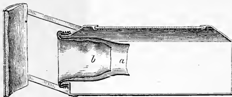
Fig. 153. — Coupe de l'appareil destiné à comprimer la main et l'avant-bras, a . — Manchon de caoutchouc invaginé dans la caisse, b . — Manchon de taffetas supprimant l'extensibilité du 1 er manchon. Une pièce retenue par des courroies empêche le bras de céder à la pression intérieure.
