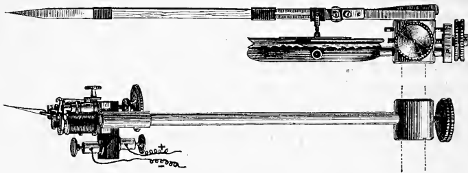
Fig. 65. — Disposition pour l'inscription simultanée du mouvement des lèvres et des vibrations du larynx.
