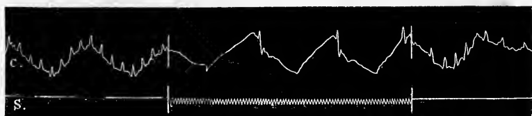
Fig. 150. — Excitations du même pneumogastrique, un peu plus bas, avec une série de secousses induites peu intenses (Bobine Du Bois).
