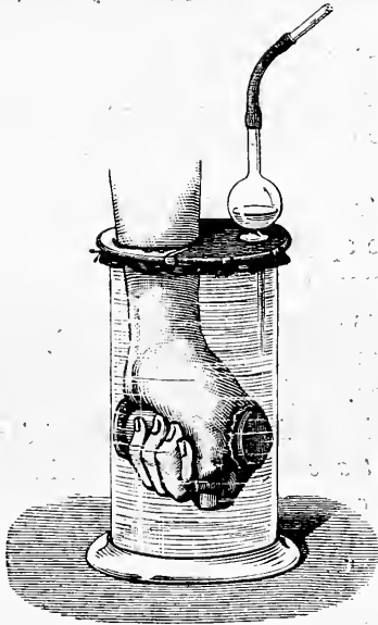
Fig. 3. — Appareil explorateur des changements du volume de la main. — La membrane au travers de laquelle passe l'avant-bras est immobilisée par une plaque métallique ; dans le tube vertical muni d'une ampoule, s'opèrent les changements de niveau qui s'inscrivent à distance à l'aide de la transmission par l'air.
