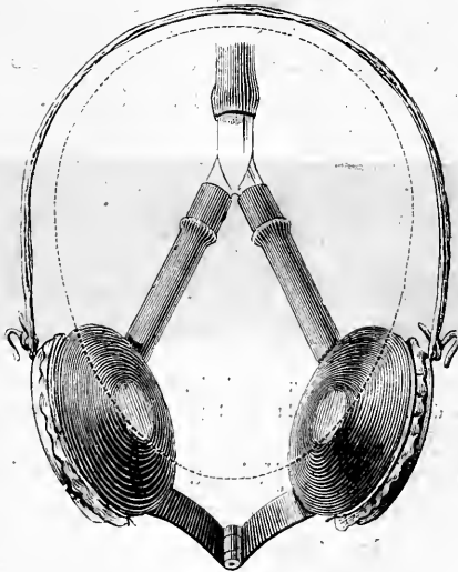
Fig. 108. — Explorateur à deux tambours conjugués pour la pulsation cardiaque des petits animaux.
