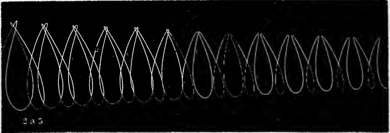
Fig. 81. — Trajectoire d'une verge de Wheatstone vibrant dans le rapport de 2 à 3; tracé recueilli sur un papier animé d'une translation rapide.
