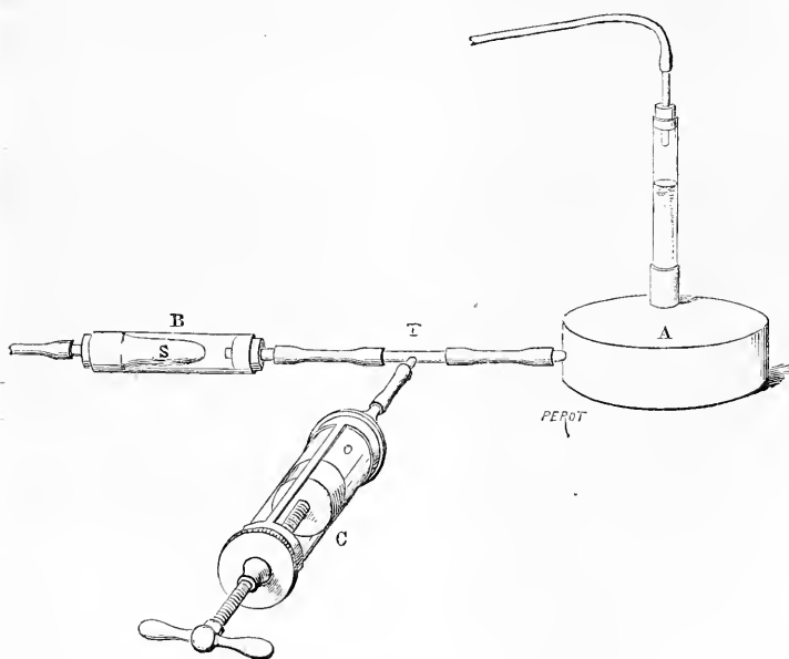
Fig. 151. — Disposition pour mesurer la pression à l'intérieur de l'ampoule S, d'après la contre-pression développée à sa surface extérieure.
