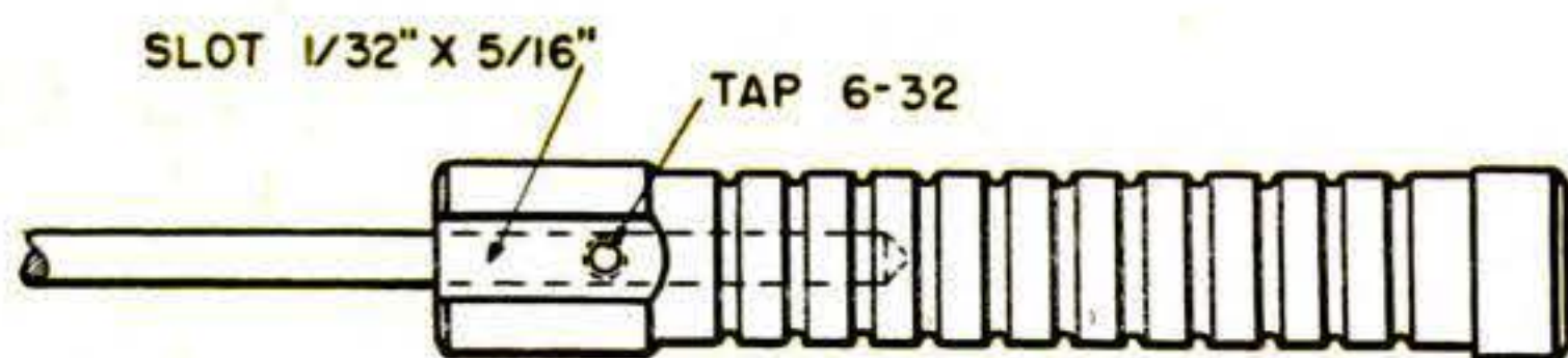
FIG. 2 HANDLE
