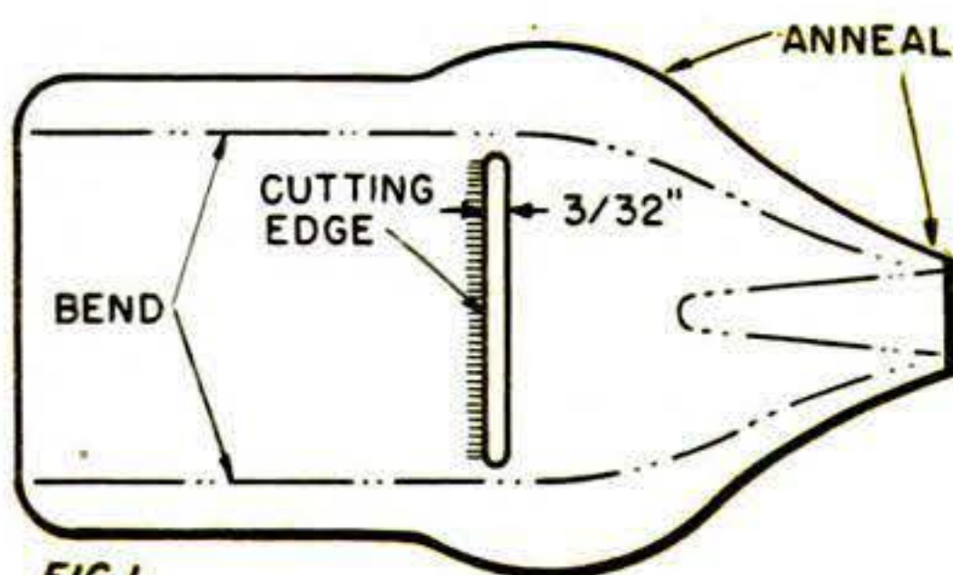
FIG. 1 KNIFE BLANK
