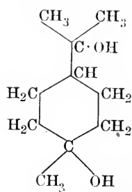
cis-Terpin.
