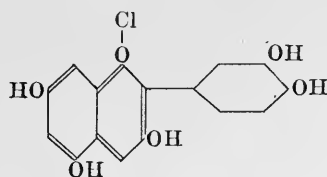
Cyanidin.
