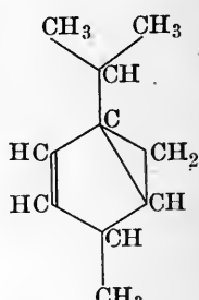
\beta -Thujene.
