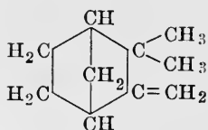
Camphene.
