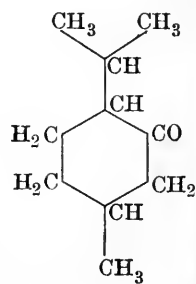
Menthone.
