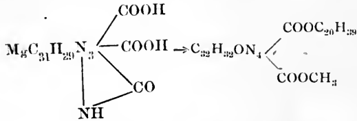
Chlorophyllin a .
