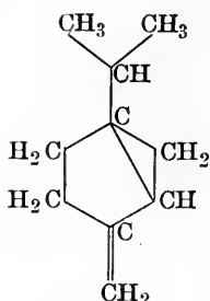
Sabinene.
