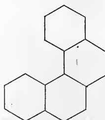
Chrysene.
