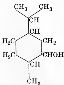
Carvomenthol.
