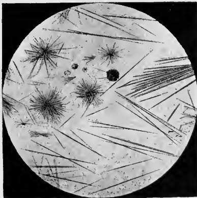
FIG. 29.—Leucine.
