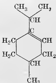
Menthene.
