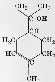
\alpha -Terpinol.
