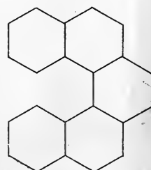
Picene.
