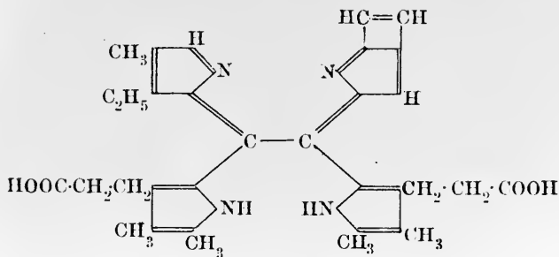
Hæmoporphyrin, \text{C}_{33}\text{H}_{38}\text{O}_4\text{N}_4 .
