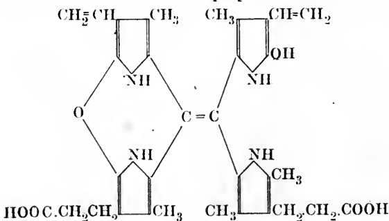
Bilirubin.
