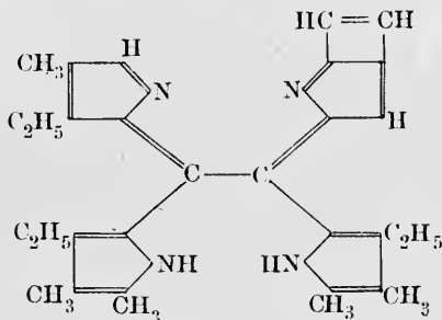
Ætioporphyrin, \text{C}_{31}\text{H}_{36}\text{N}_4 .
