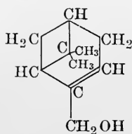
Myrtenol
