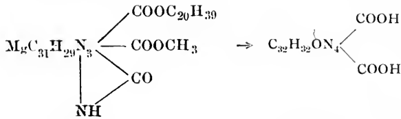
Chlorophyll a .
