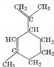
\gamma -Terpinene.
