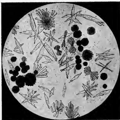
FIG. 49.—Sodium urate. (After Funke.)
