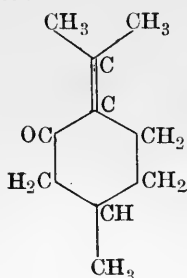
Pulegone.
