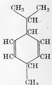
2, 4- \Delta -Menthadiene, not natural.
