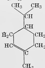
Carvomenthene.
