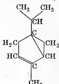
\alpha -Thujene.
