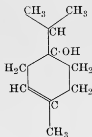
Terpinenol.
