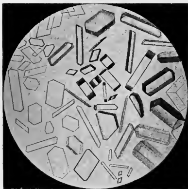
FIG. 28.—Glycine.
