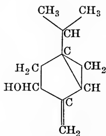
Sabinol.
