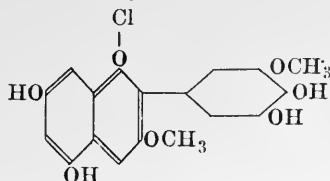
Oenidin.
