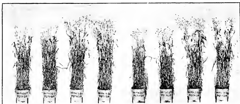
Fig. 10.—Effets de la potasse sur l'avoine.
