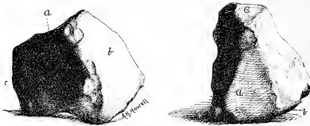
DE CEWSVILLE METEORITE.
