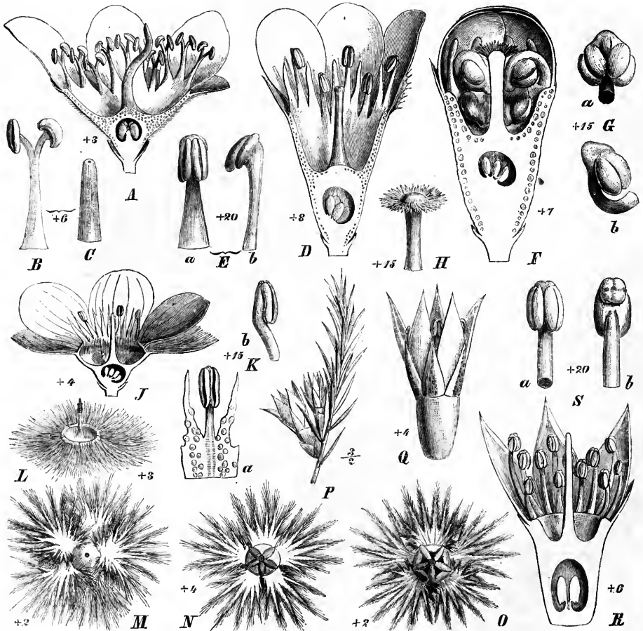
Fig. 49. A-C Pileanthus Limacis Lab. A Bl. längs durchschnitten; B Stb.; C Gr. — D Bl. längs durchschnitten und E Stb. ( a von vorn und b von der Seite) von Chamaelaucium ciliatum Desf. — F-H Ch. uncinatum Schau. F Knospe längs durchschnitten; G Stb., a von vorn, b seitlich; H Gr. — J-L Verticordia picta Endl. J Bl. längs durchschnitten; K Stb., a von vorn mit 2 Staminodien, b von der Seite; L Kelch und Gr. — M Kelch von V. Cunninghamii Schau., von unten gesehen. — N desgl. von V. Drummondii Schau. — O desgl. von V. chrysostachya Meißn. (die äußeren Kelchb. abgeschnitten). — P-S Homalocalyx ericaeus F. v. Müll. P Zweig mit Bl.; Q Bl.; R Bl. längs durchschnitten; S Stb., a von vorn, b von hinten. (Original.)
