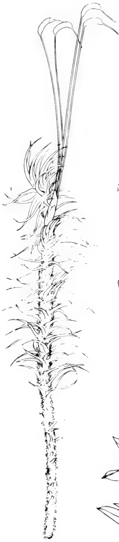
Dicranum polysetum
