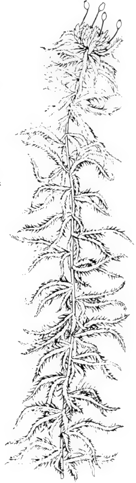
Sphagnum cuspidatum
