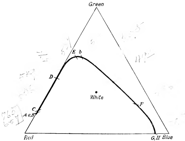
Fig. 8. Colour triangle. A, B, C, etc., Fraunhofer lines. (König.)
