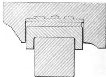
Section A-B.
