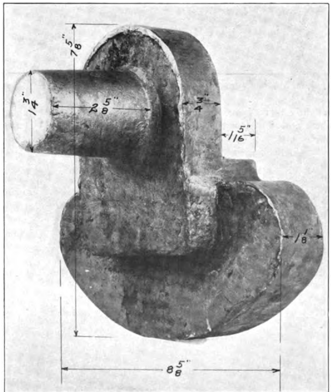
Fig. 3—Link Trunion
