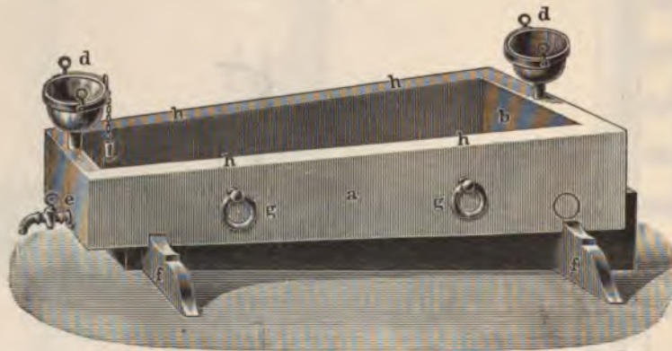
a Metallwanne; b Rückwand, welche noch mit einem schrägen Brett für den Kopf versehen wird; d Trichter zum Füllen der Doppelwände; e Auslasshahn; f Füße; g Handhaben zum Transport der Wanne.
