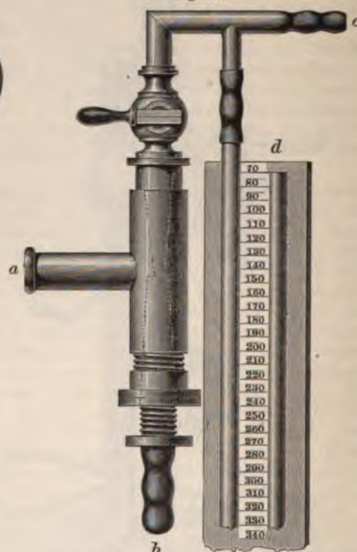
Wasserstrahlsaugpumpe. a Wasserzuluß, b Wasserabfluß, c Luftsangrohr, d Barometer.
