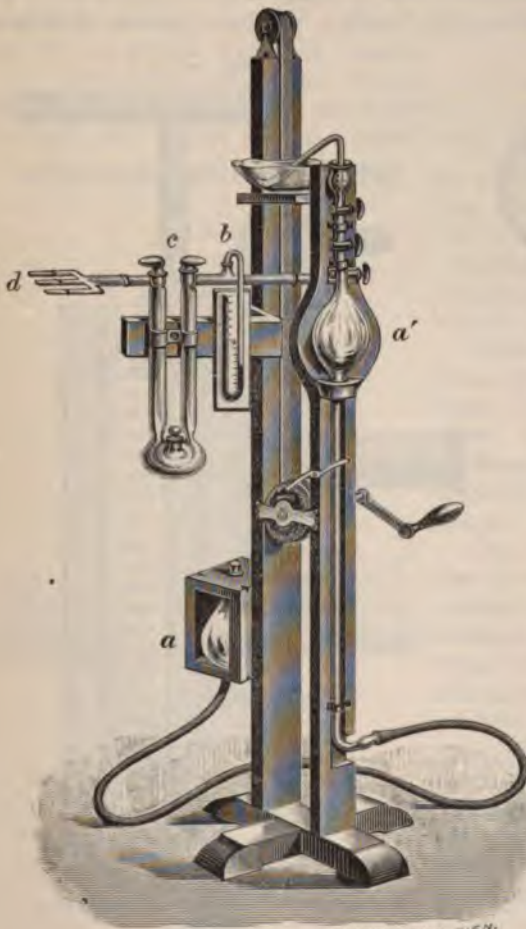
a' Glaskugeln, b Barometer, c Trockenapparat, d S Rohre zum Anschluss an Recipienten.
