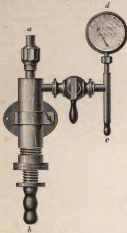
Wasserstrahlsaugpumpe. a Wasserzuluß, b Wasserabfluß, c Luftsangrohr, d Aneroidbarometer.
