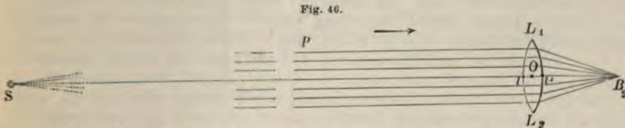
Fig. 46. S ist der ferne Lichtpunkt. Um anzudeuten, dass S im Verhältnis zu den Ausdehnungen der Zeichnung ausserordentlich weit von der Linse L_1 L_2 entfernt zu denken, ist der Anfang des von S ausgehenden Strahlenbündels punktiert. Der Pfeil giebt die Richtung der Strahlen.
