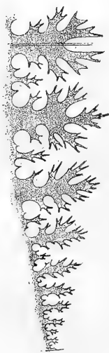
Phylloceras semisulcatum , d'après d'Orbigny (pl. LIII, fig. 6).
