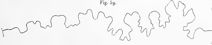
Sphenodiscus Requieni (gros. = 3,7), d'après un échantillon des environs de Tours.
