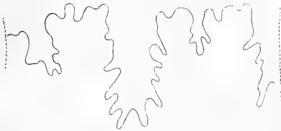
Am. Bourgeoisi (gros. = 4).
