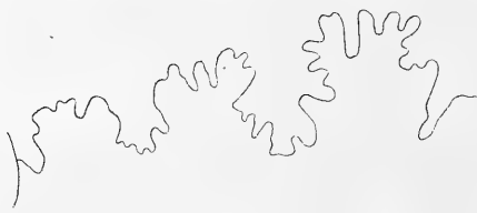
Barroisia Haberfellneri (gros. = 3,5), dessin de M. Douvillé, d'après l'échantillon représenté pl. II, fig. 3.
