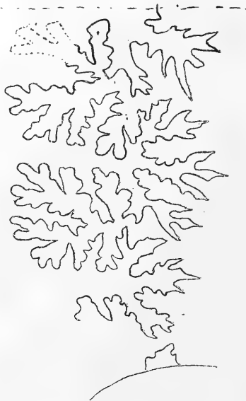
Pachylidiscus Sturti (gros. = 5), d'après un échantillon de Gan.
