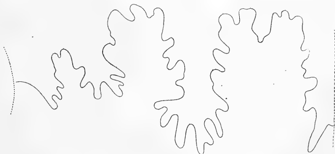
Gauthiericeras Margæ (gros. = 3,3), d'après l'échantillon représenté pl. XV, fig. 2.
