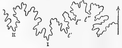
Sonneratia Cleon (gros. = 4,5), d'après Douvillé, B. S. G. F., 3 e , XVIII, p. 289.
