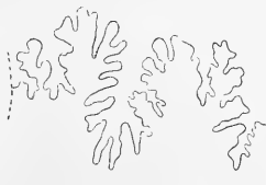
Peroniceras Mouretii (grand. nat.), d'après un échantillon de la craie de Villedieu.
