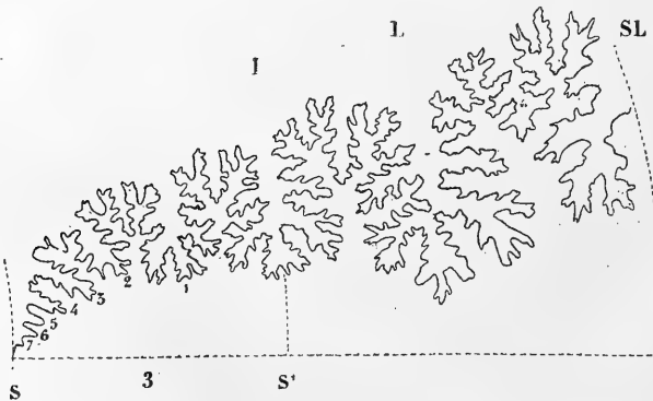
Desmoceras Stobæi , d'après Moberg, Cephalopoderna... (Pl. II, fig. 3).
