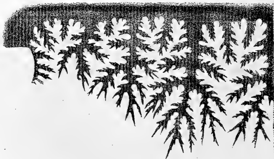
Pachydiscus neubergicus , d'après Seunes, pl. II, fig. 2 o .
