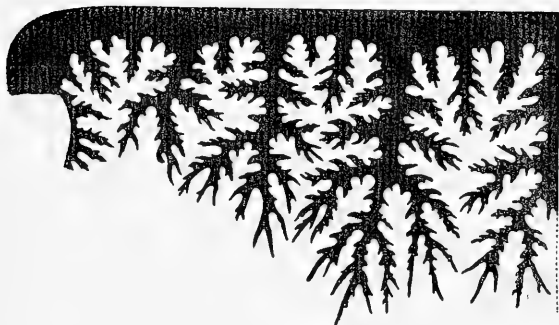
Pachydiscus neubergicus , d'après Seunes, pl. II, fig. 2°.
