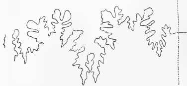
Ancyloceras (?) Douvilléj (gros = 3), d'après l'échantillon représenté pl. XXXV, fig. 8.
