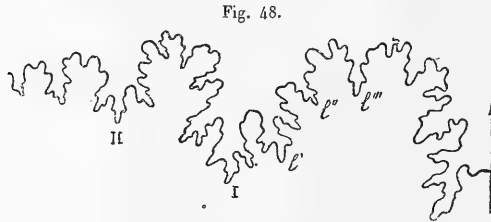
Hoplites splendens (gros. = 4,5), d'après Douvillé, B. S. G. F., 3 e , XVIII, p. 289.
