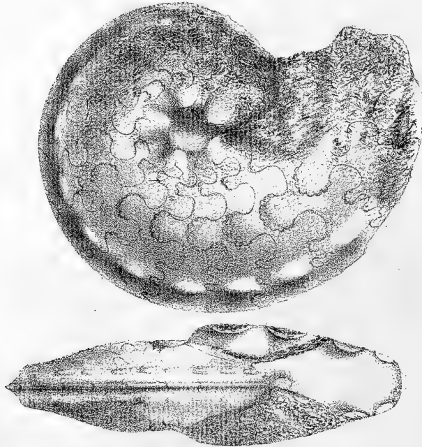
Tisotia Slizewiczi , reproduction de la figure donnée par M. Fallot, Crétacé. . . . pl. II, fig. 2.
