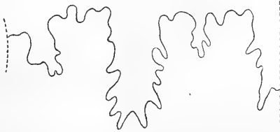
Mortoniceras Bourgeoisi (gros. = 4), d'après l'échantillon de la craie de Villedieu représenté pl. XIV, fig. 5.
