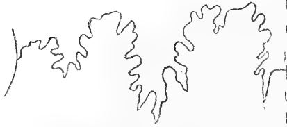
Schlönbachia varians (gros. = 5), d'après un échantillon de Rouen.
