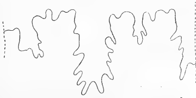
Mortonicerat Bourgeoisii (gros. = 4), d'après l'échantillon de la craie de Villedieu représenté pl. XIV, fig. 5.
