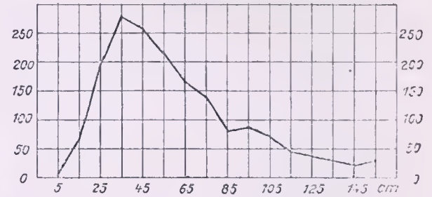
Abb. 3. Verteilung von 775 Gemälden nach der Breite der Bilder.
