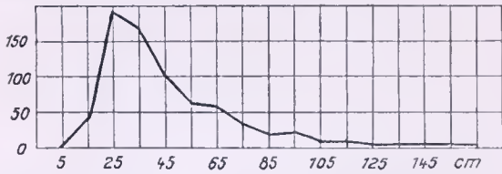
Abb. 3. Verteilung von 775 Gemälden nach der Breite der Bilder.
