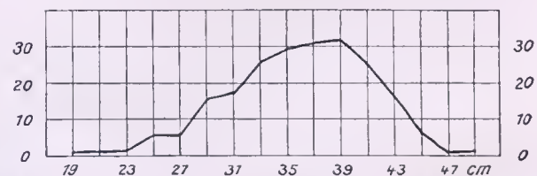
Abb. 2. Verteilung der Längen des zweiten Gliedes von 217 Roggenhalmen.
