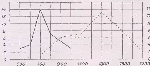
Abb. 8. Verteilungskurve der Leistung einer Schullasse im Rechnen (Addieren einstelliger Zahlen) vor und nach systematischer Übung.
