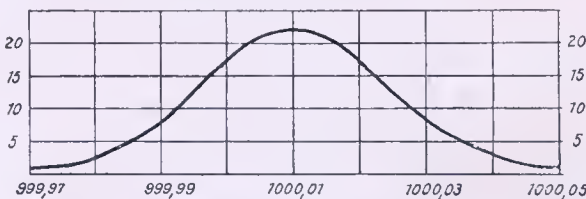
Abb. 1. Verteilungskurve beim achzigmaligen Messen eines Stabes.
