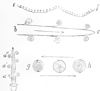
FIG. 1. Vortici grandinosi.
