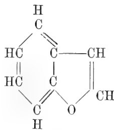
Cumarone
