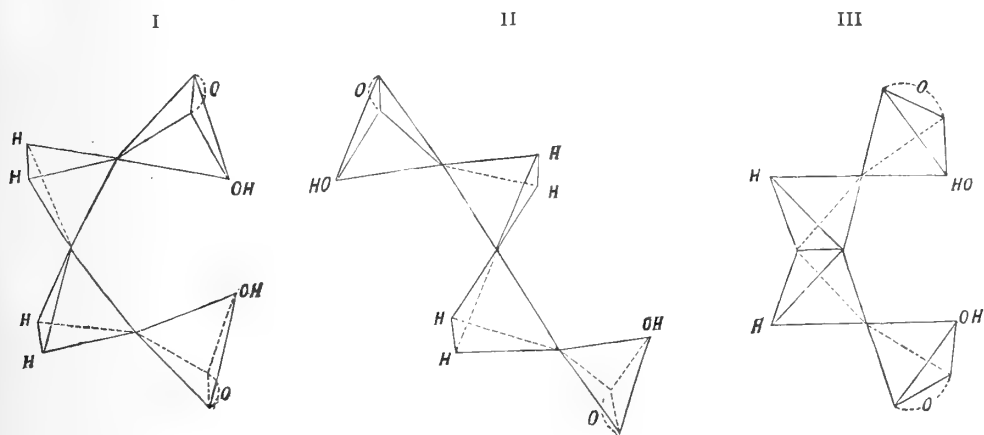
Acido succinico nella posizione maleica.
