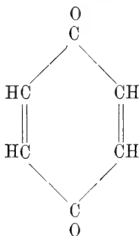
Chinone.
