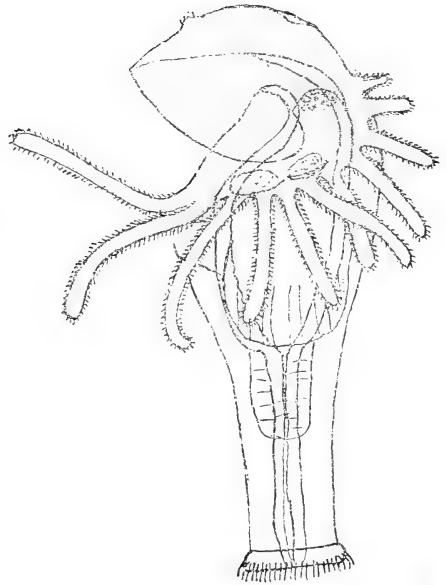
PHORONIDEA.—FIGURE I.
